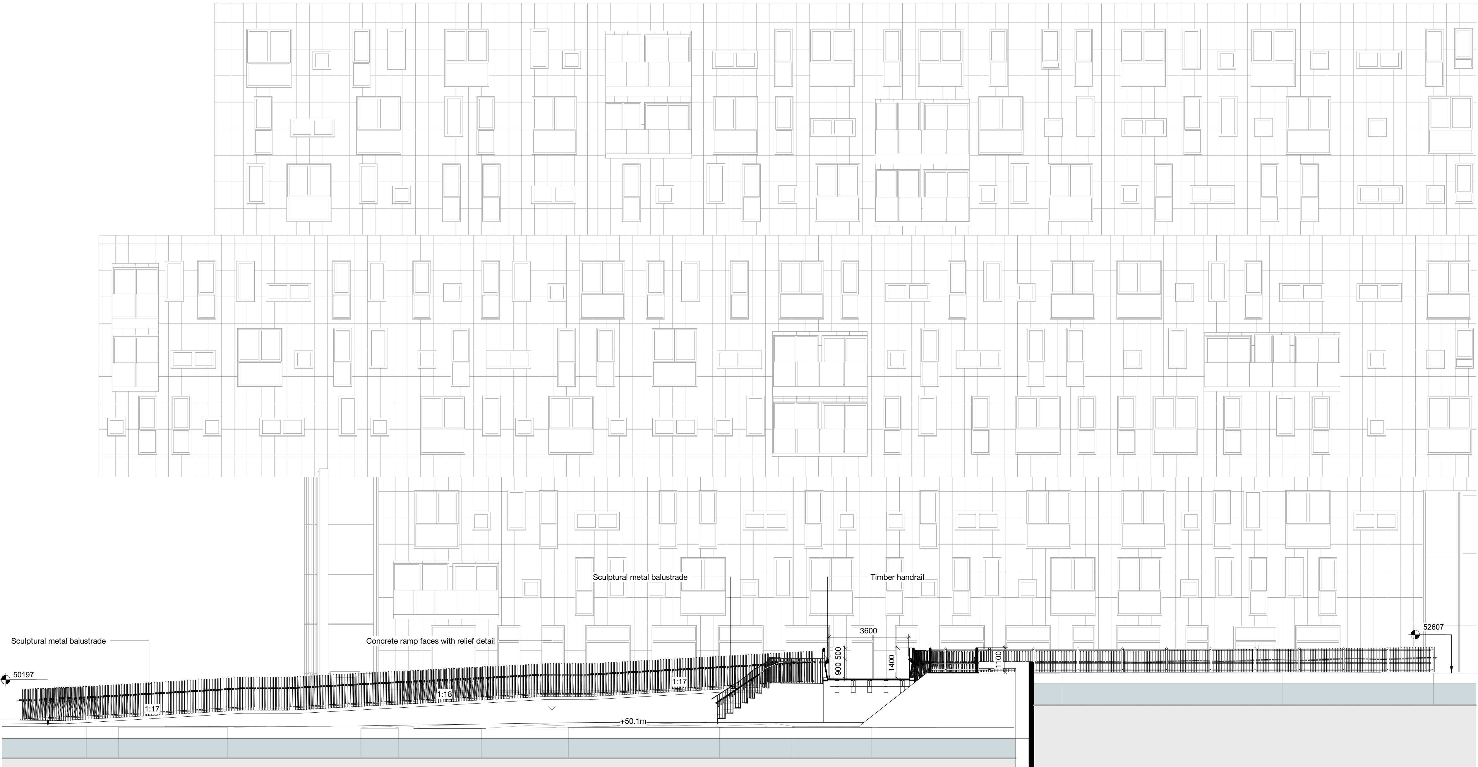
Elevation A-A 1 : 100
