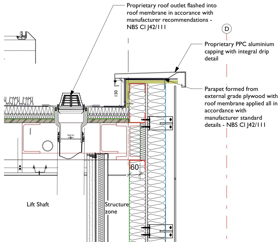
2 Parapet/Drainage Outlet Scale: 1:10
