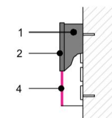
PINK APOSTROPHE (') CROSS SECTION SCALE : N.T.S.
