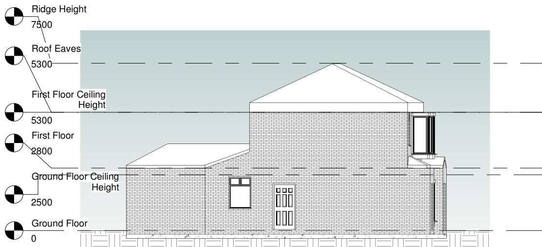
2 East 1 : 100
