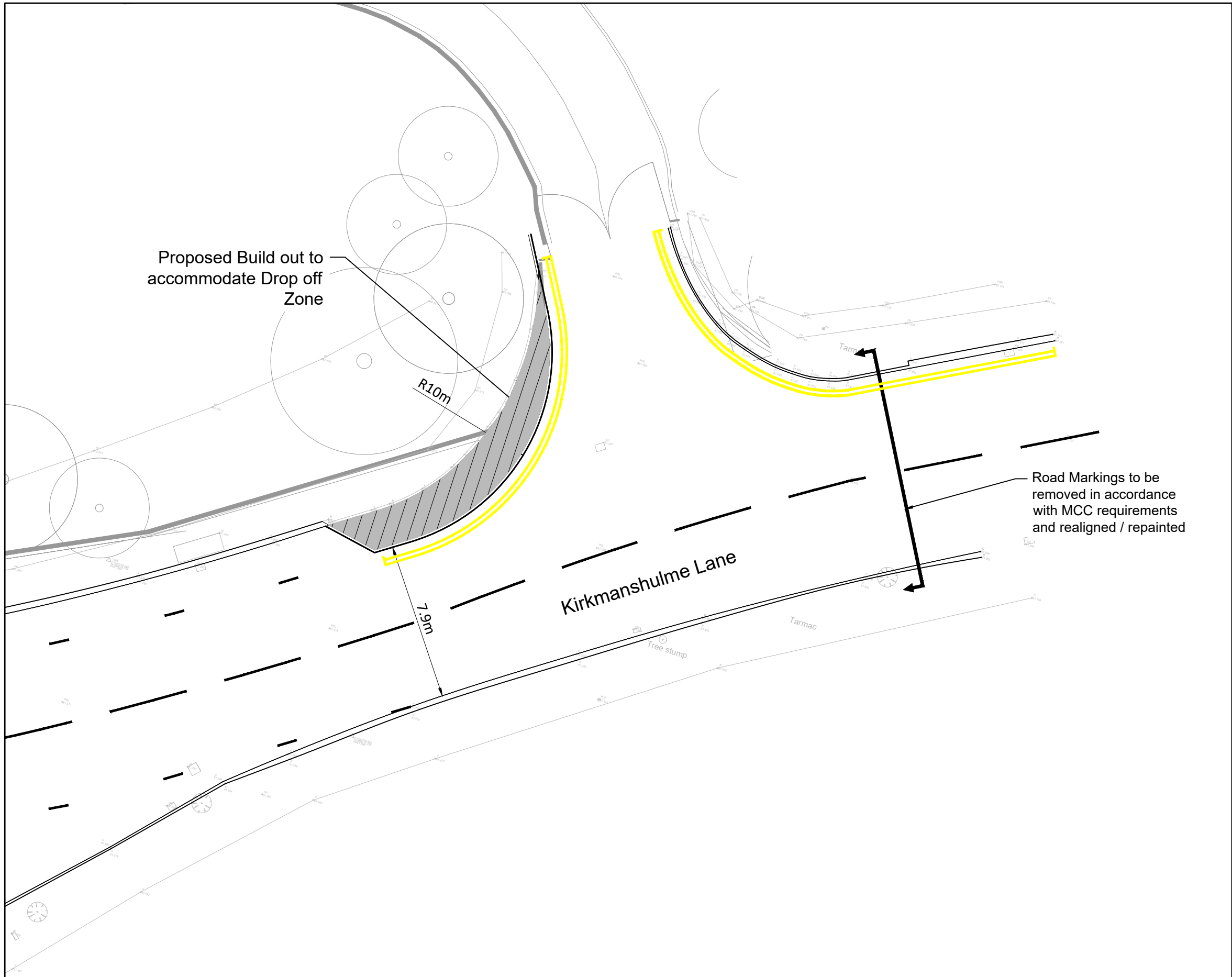
Inset 2 Scale 1:200
