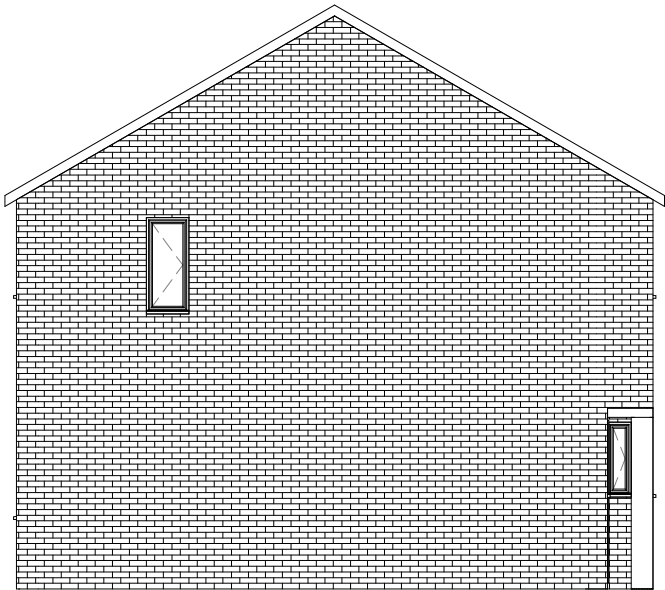
2 Left Existing 1 : 100
