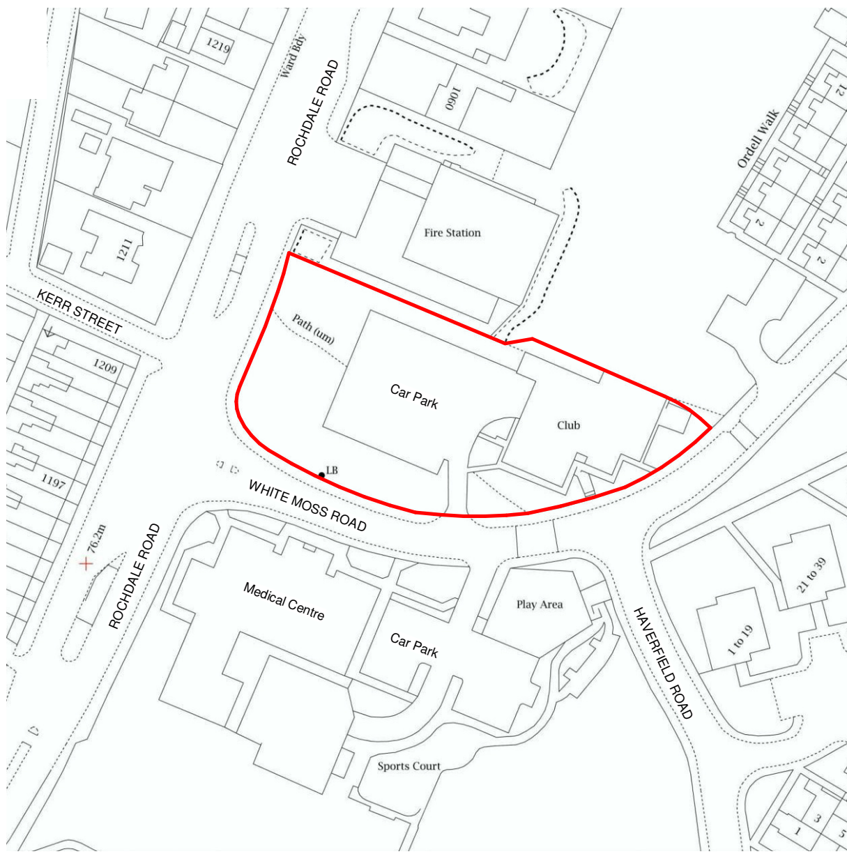
Site Location 1 : 1250
