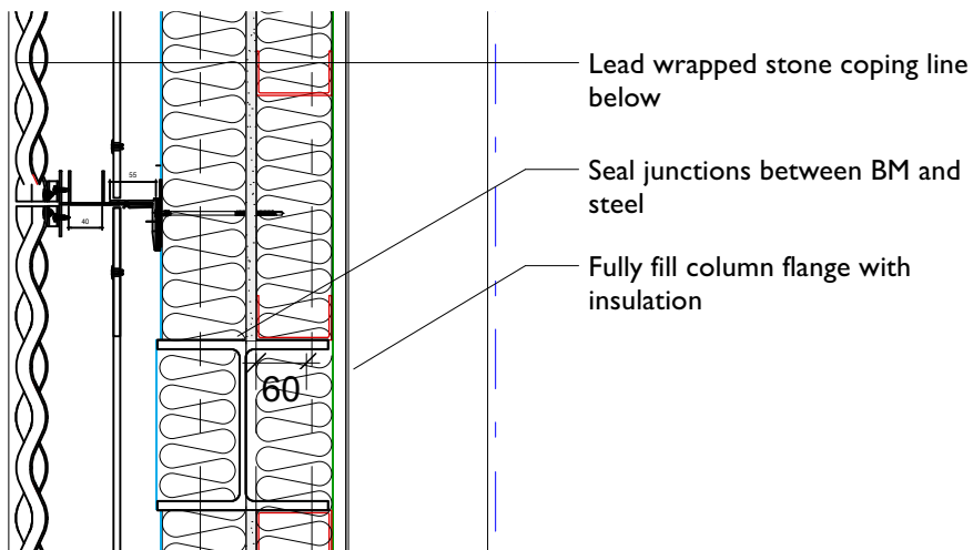
3 Plan Detail - Parapet Scale: 1:10
