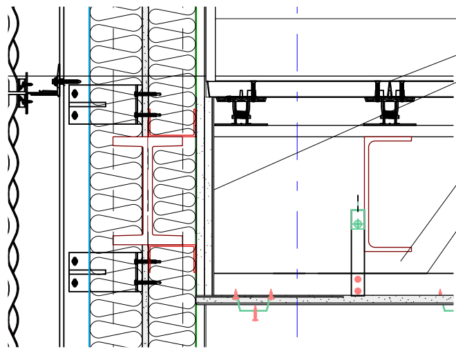
1 Floor Edge Scale: 1:10
