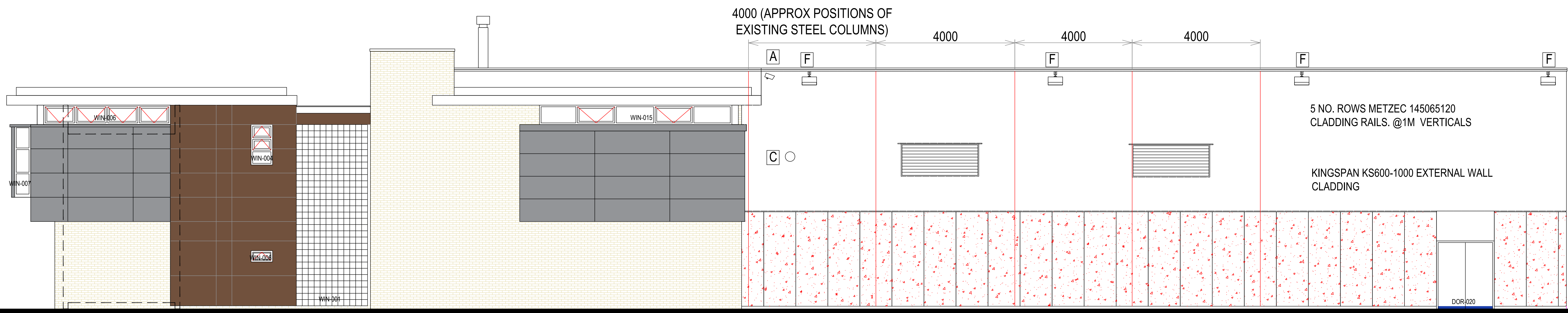
Elevation 4
