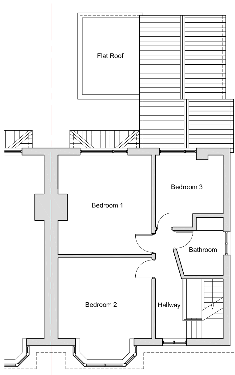
Existing 1/F Plan 1:100
