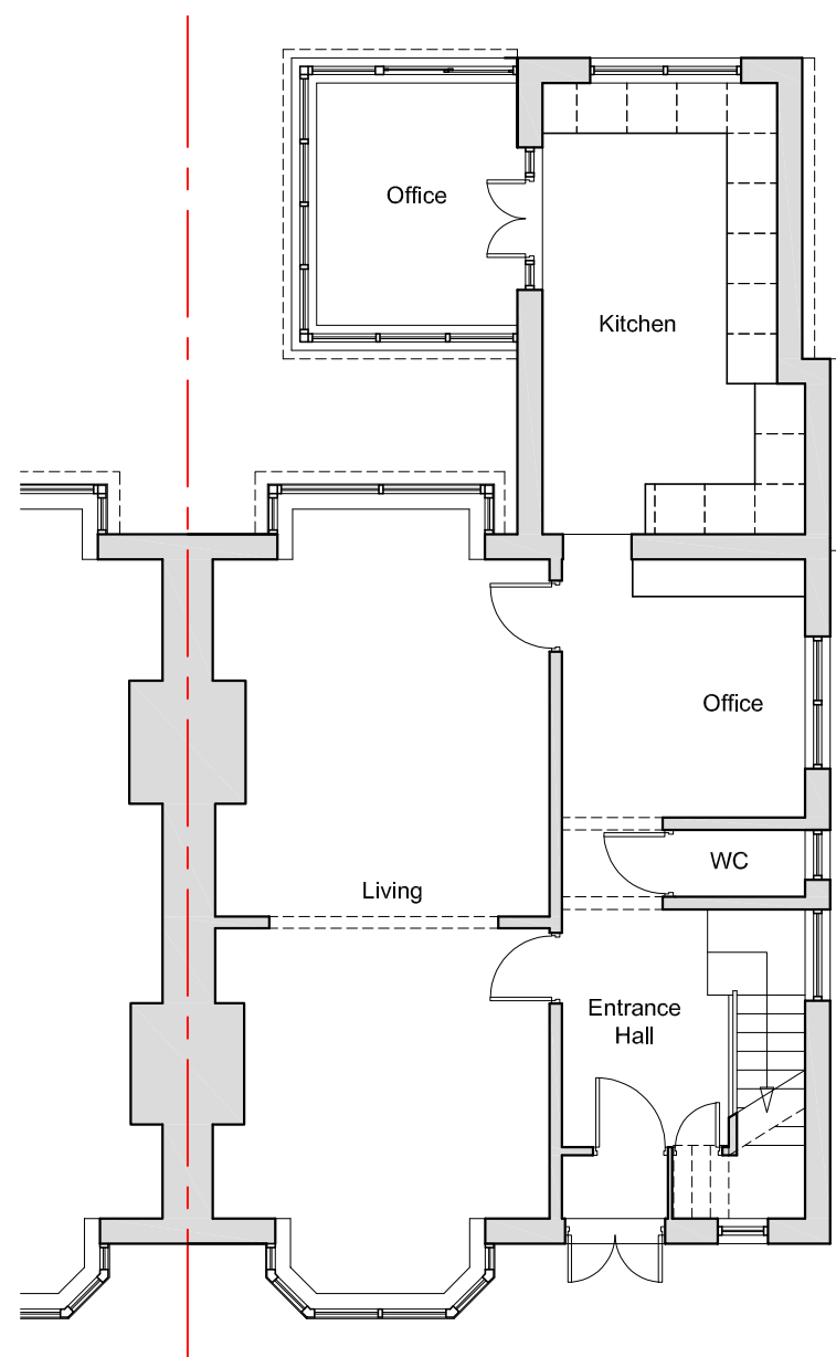
Existing G/F Plan 1:100
