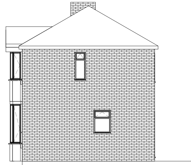
4 Right Existing 1 : 100
