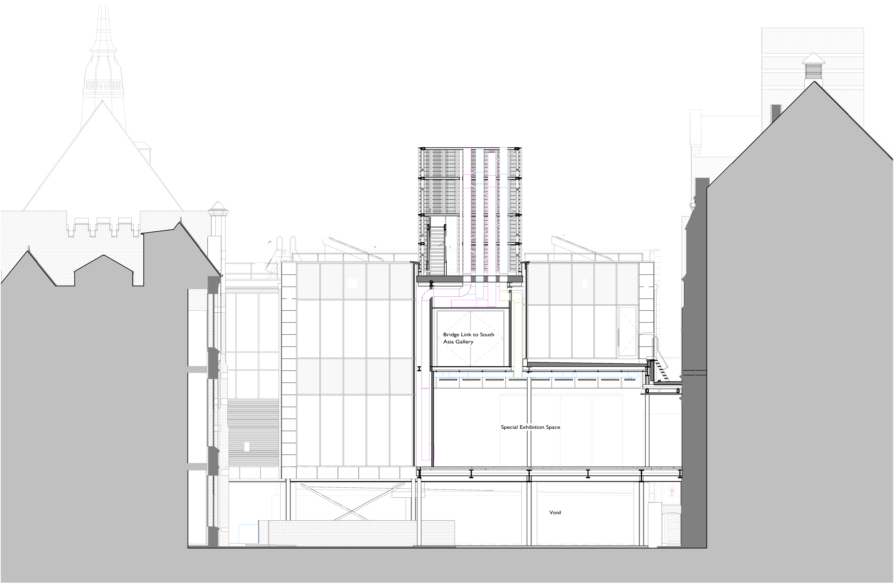
1 Existing Section GG 231 1 : 100
