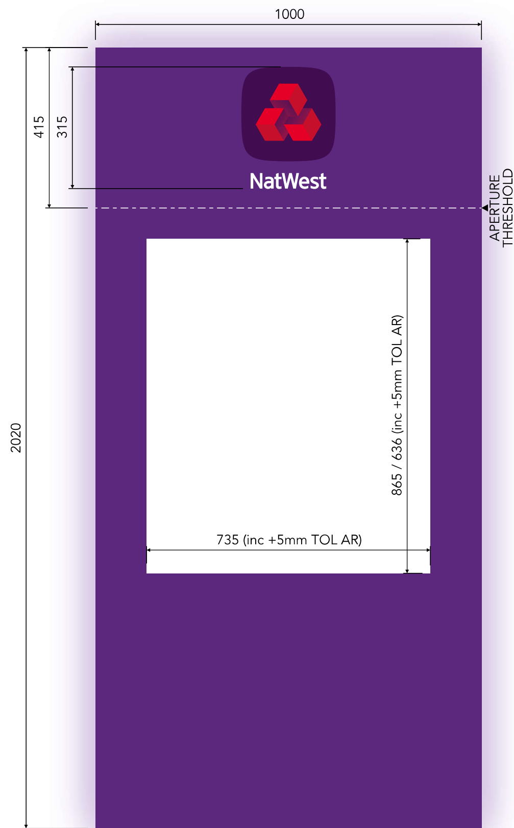
FACE 1:10
