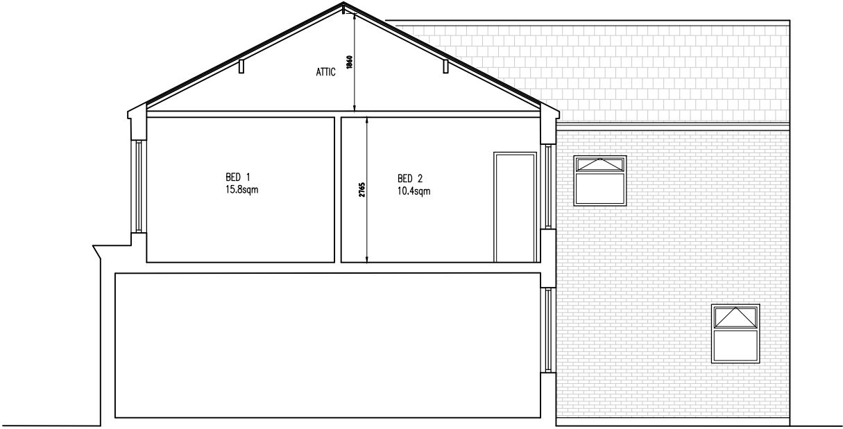
EXISTING SECTION A-A 1:100 @ A3
