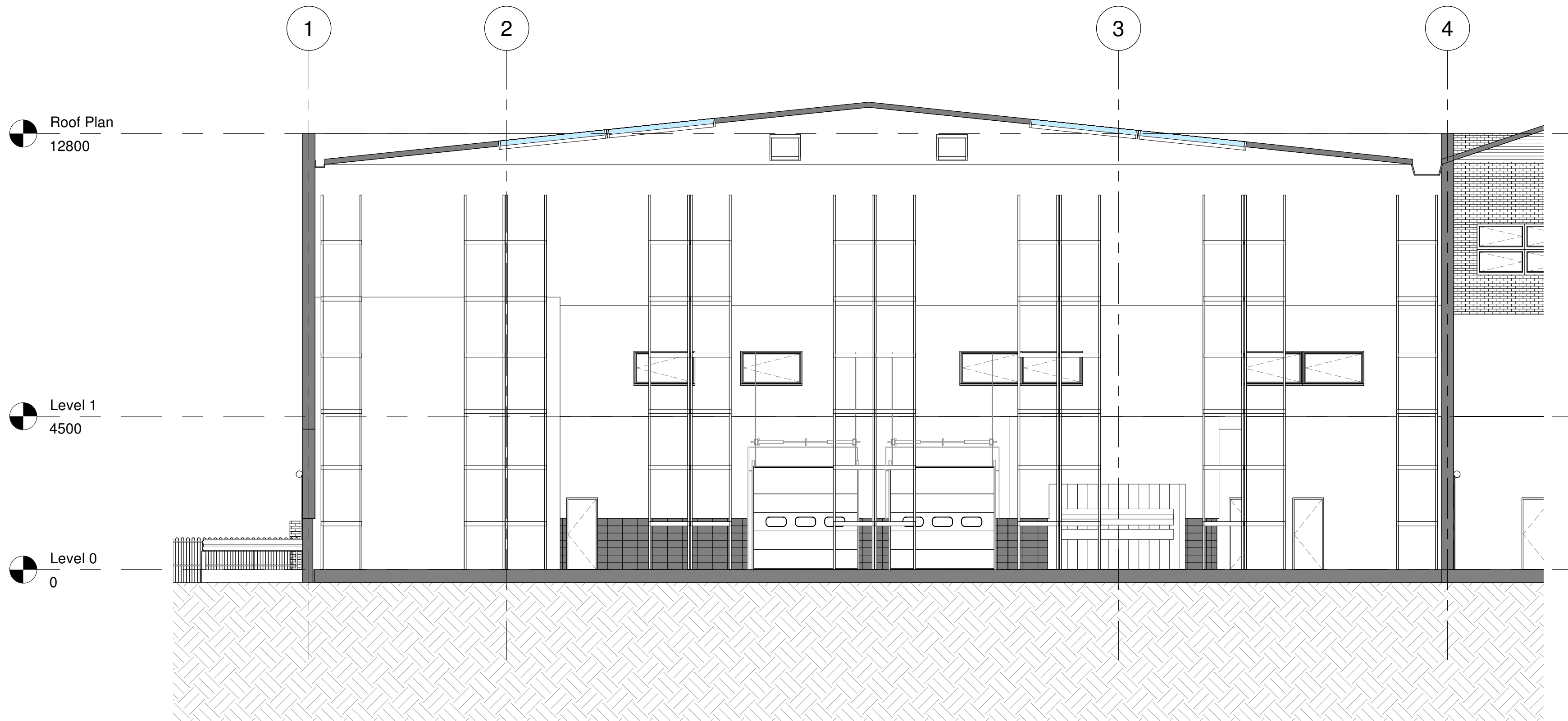
2 Section A 1 : 100
