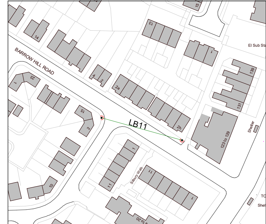
1. Site - LB11 - Location Plan 1 : 1250
