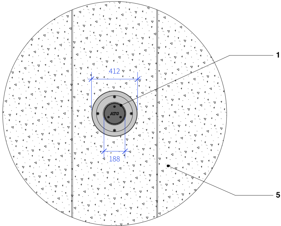
Retractable Bollard RB2 - Plan Scale: 1:20
