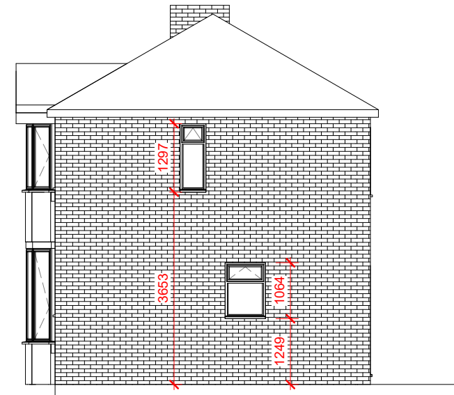
4 Right Existing 1 : 100
