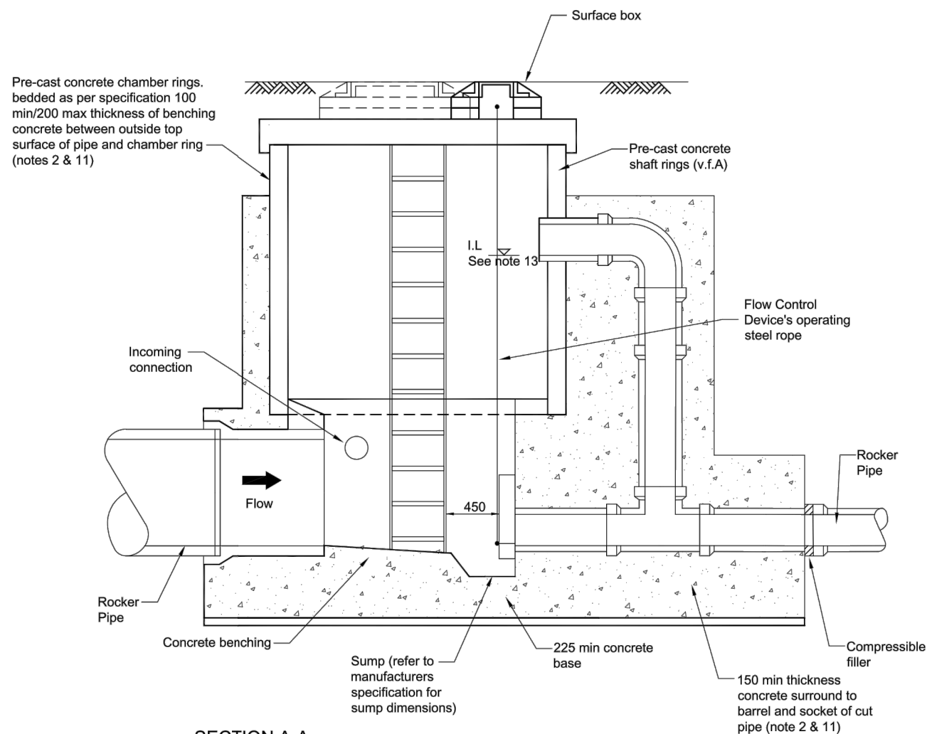
SECTION A-A
