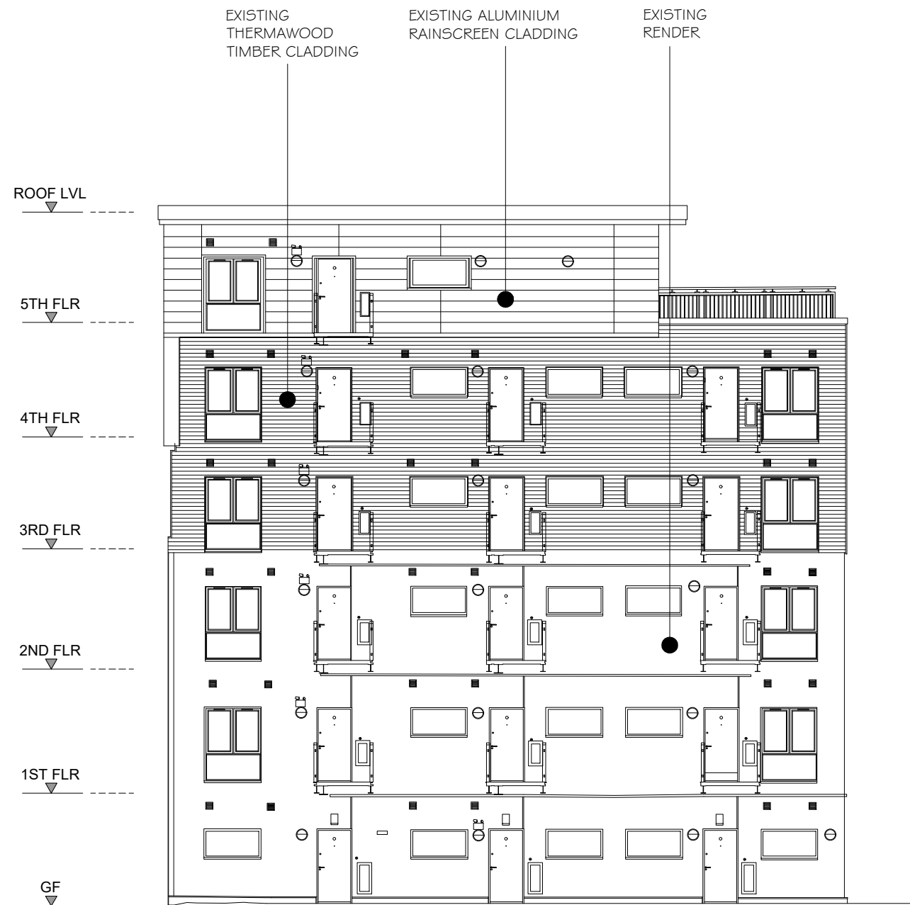
ELEVATION 3
