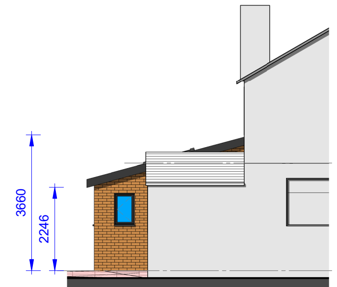
02-P-Elevation 1 : 100
