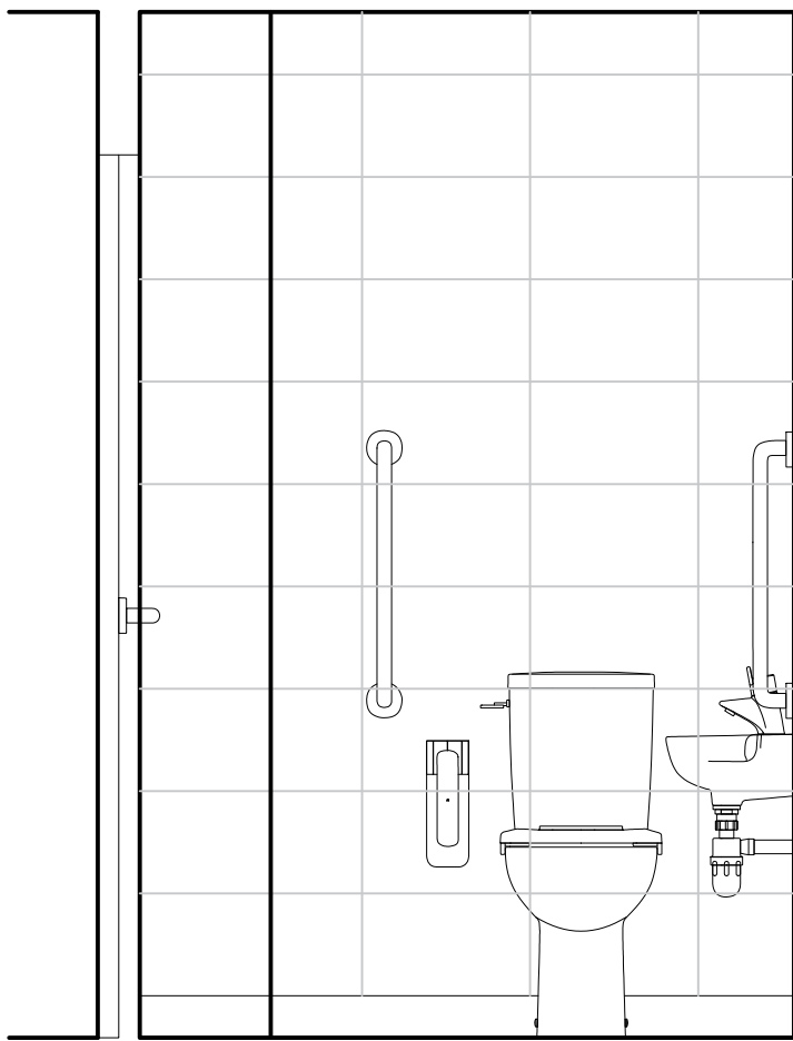
ELEVATION A-A
