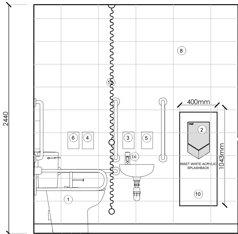
ELEVATION B-B
