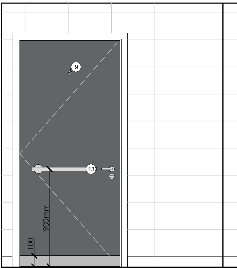
ELEVATION D-D
