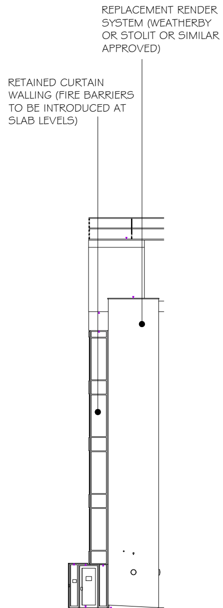
ELEVATION 12
