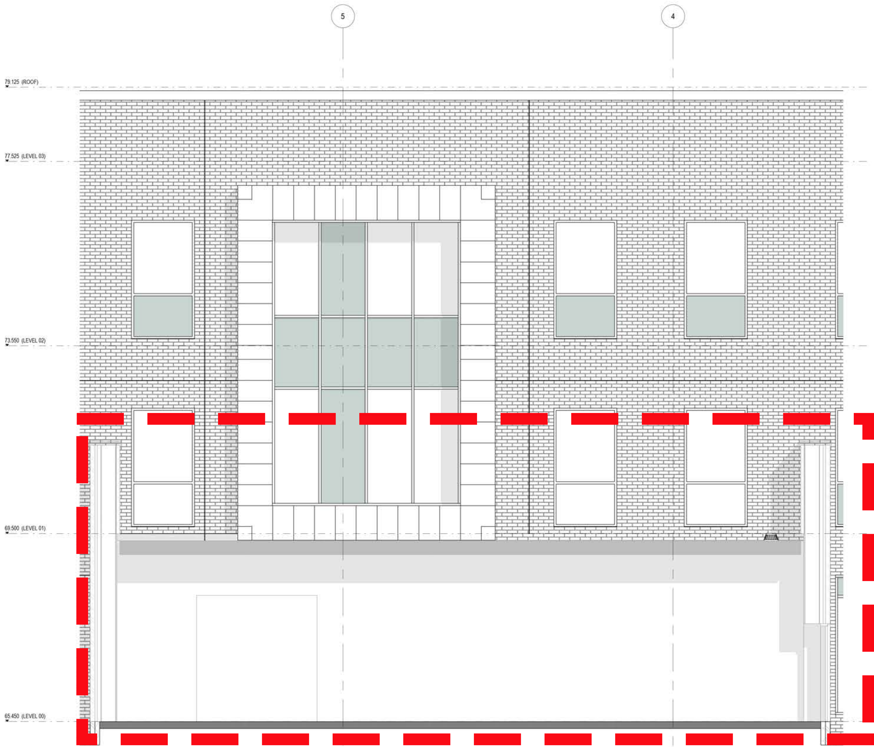
3 Elevation 1 - a 1:50
