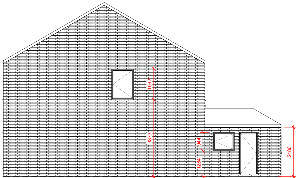
4 Right Existing 1 : 100
