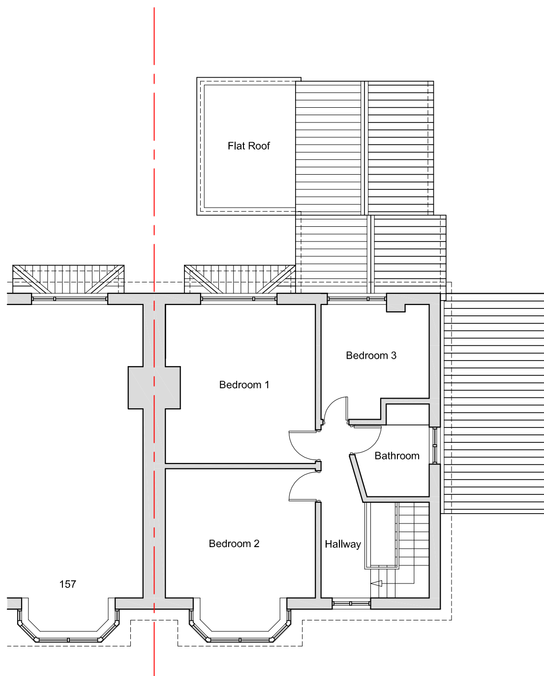
Existing 1/F Plan 1:100
