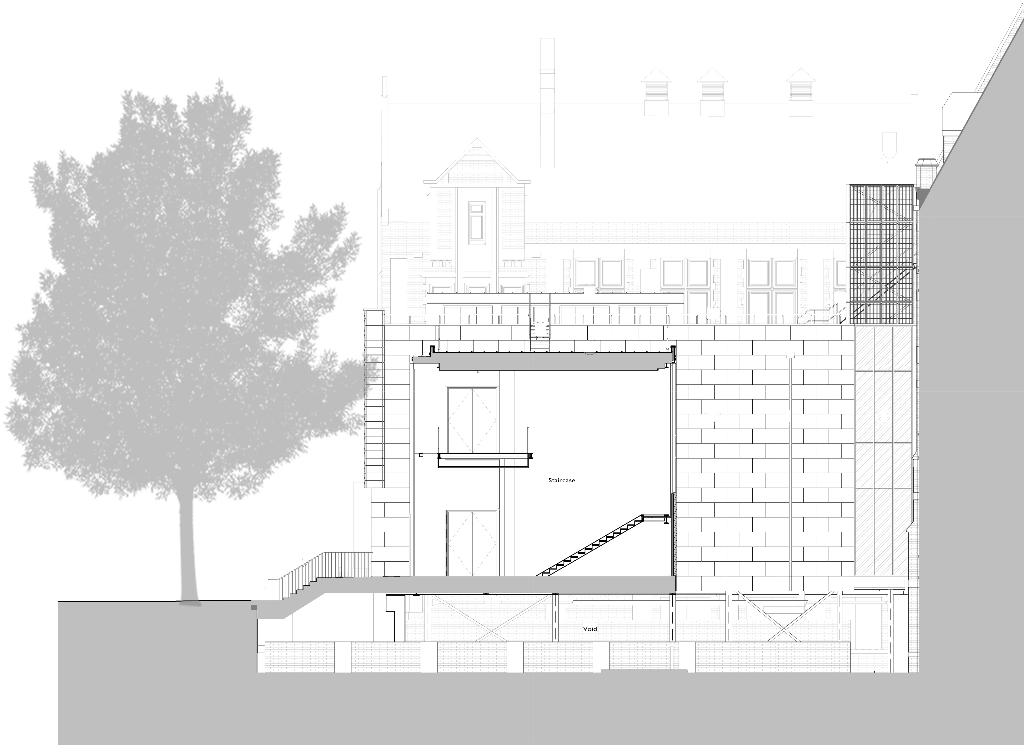
1 Existing Section BB 226 1 : 100
