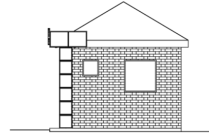
RIGHT ELEVATION
