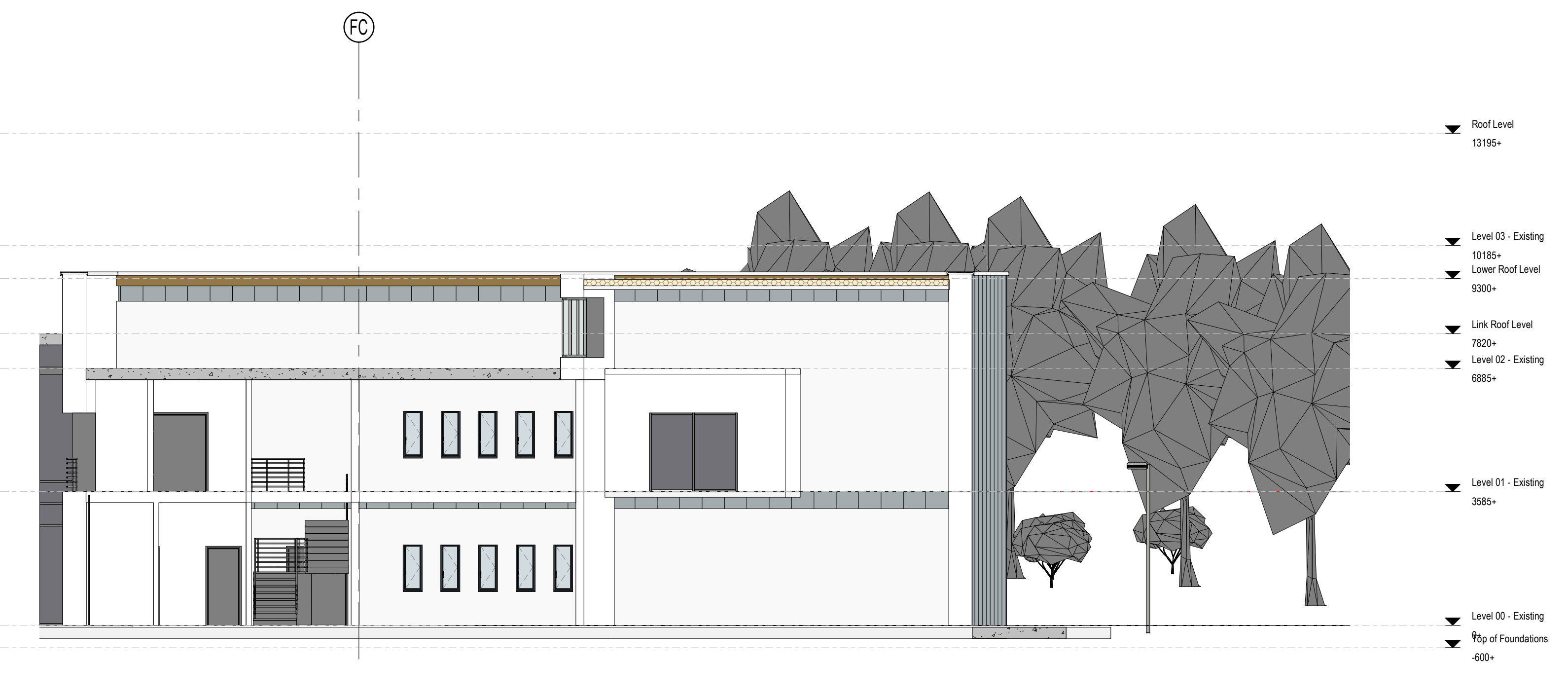
2 | (06)_SectBB Existing
