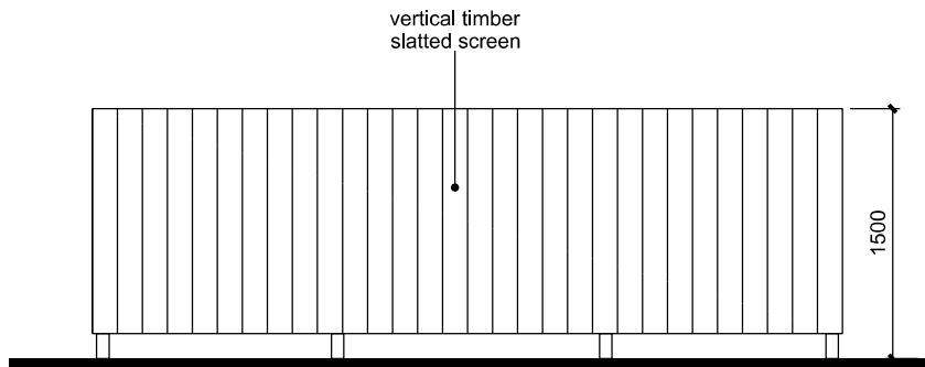
Elevation 01 & 03
