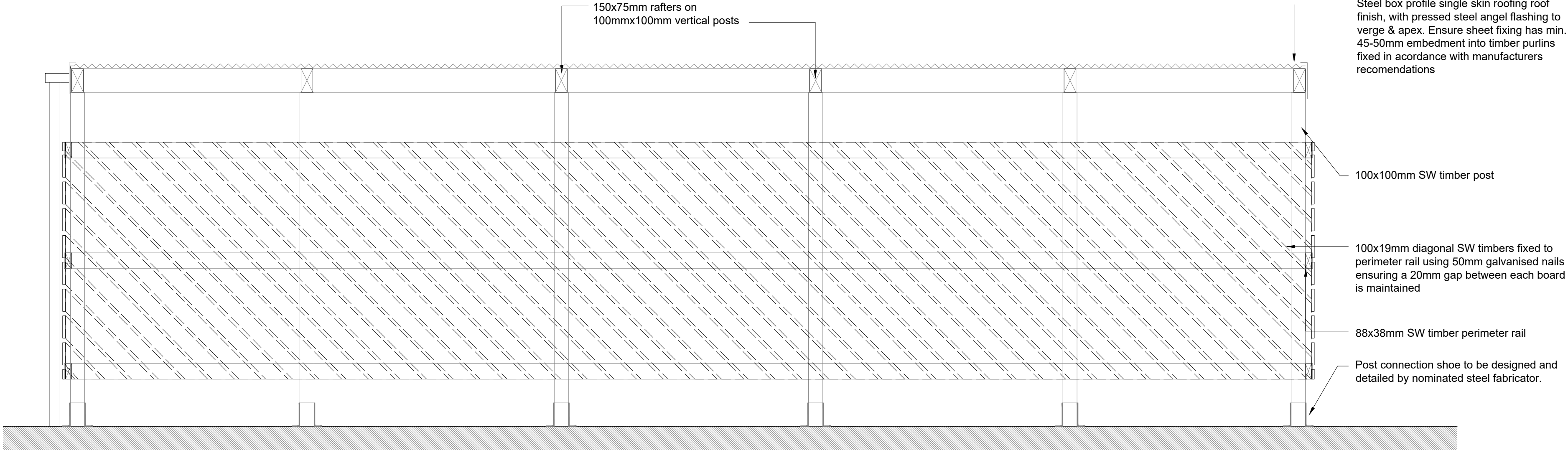
SECTION A-A SCALE 1:20
