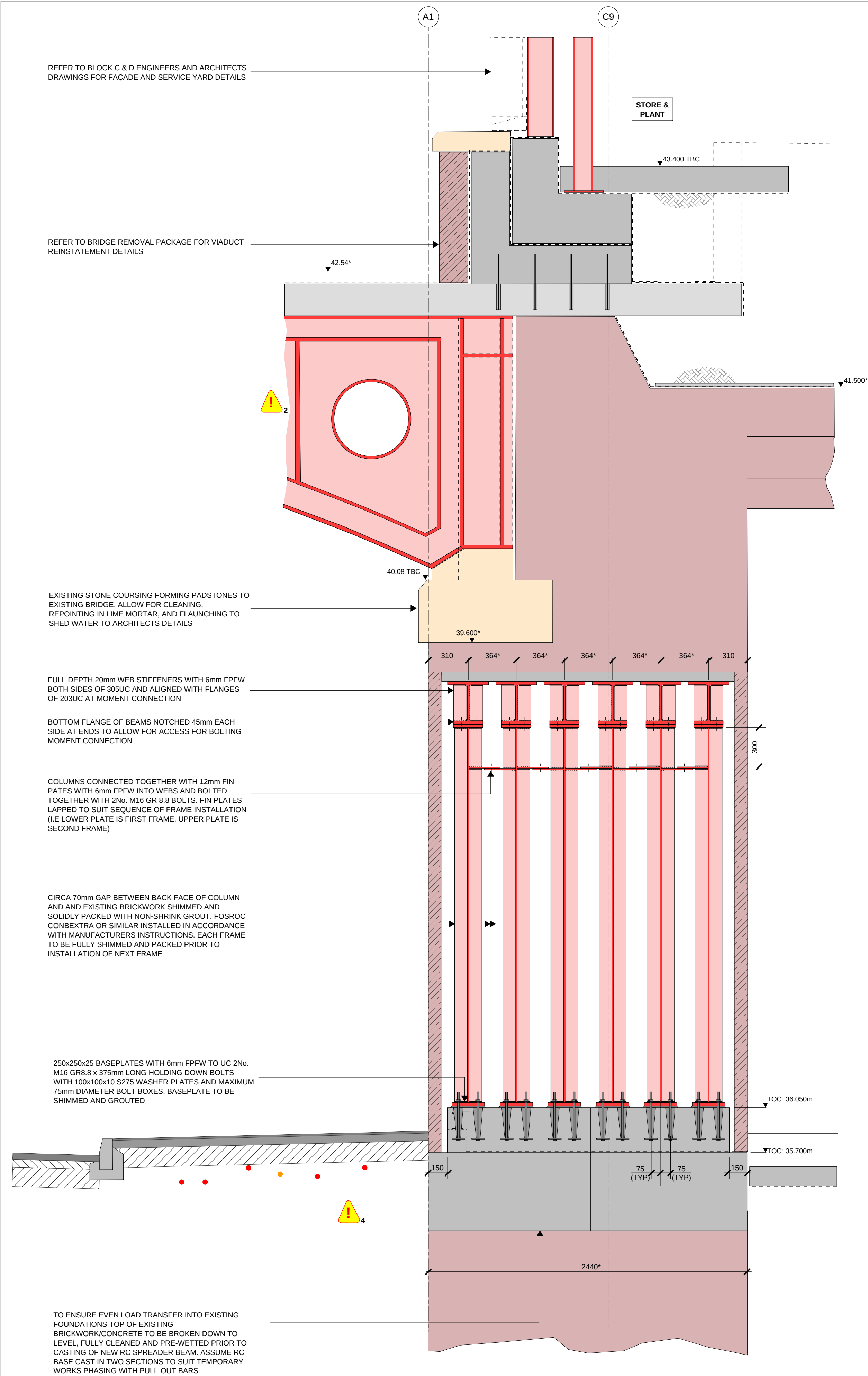
SECTION A-A 1:20
