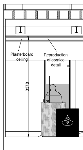
Section F 1:20 @ A1 1:40 @ A3
