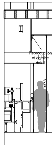
Section E 1:20 @ A1 1:40 @ A3
