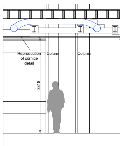
Section G 1:20 @ A1 1:40 @ A3
