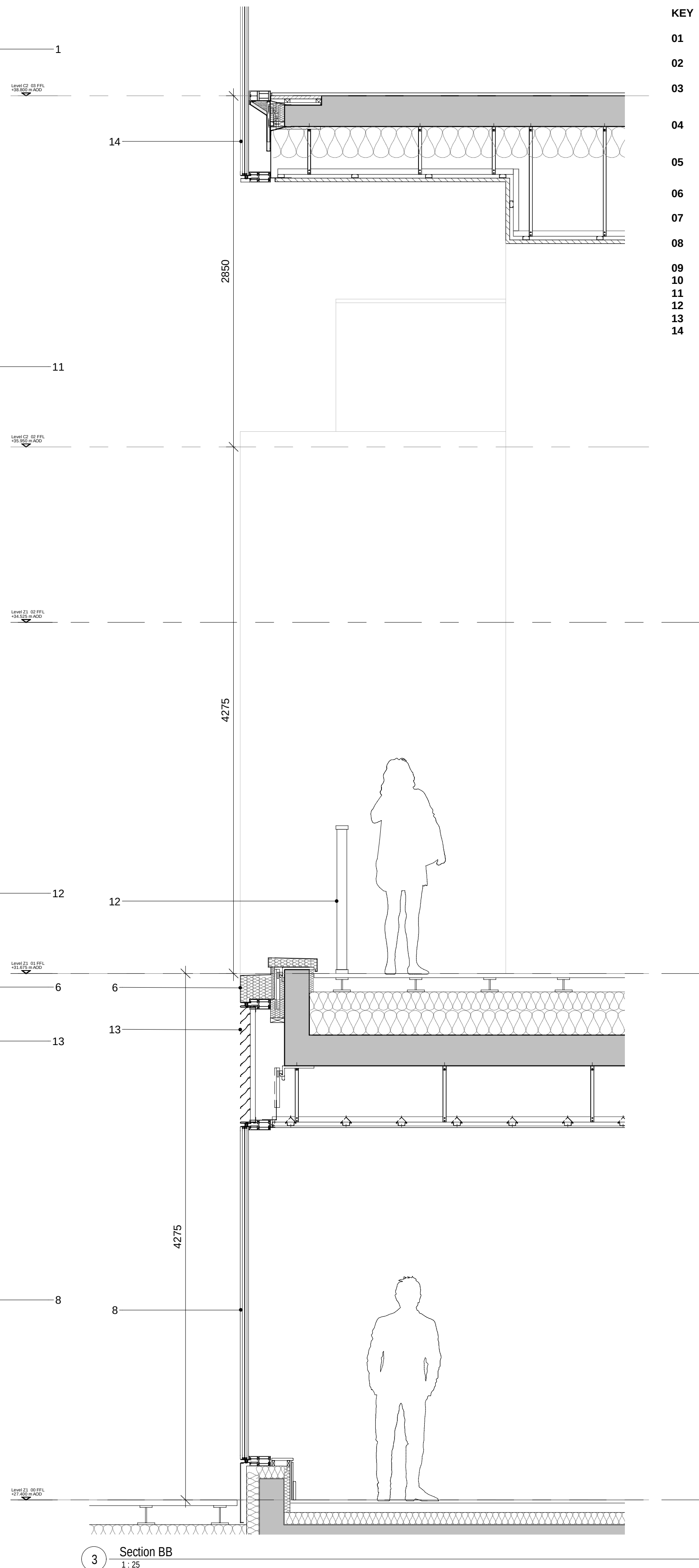
3 Section BB 1:25
