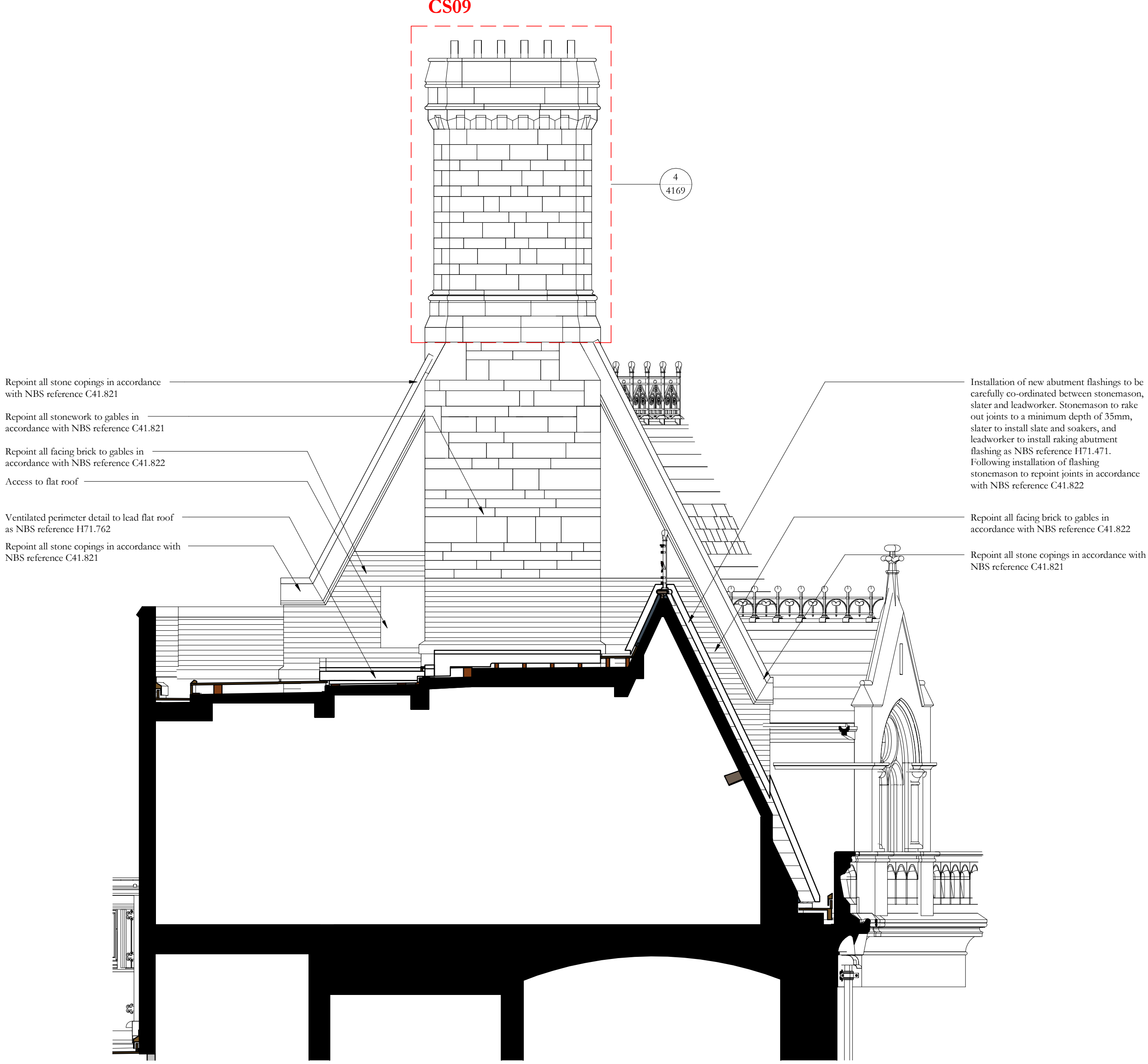
Section BU 1 : 50
