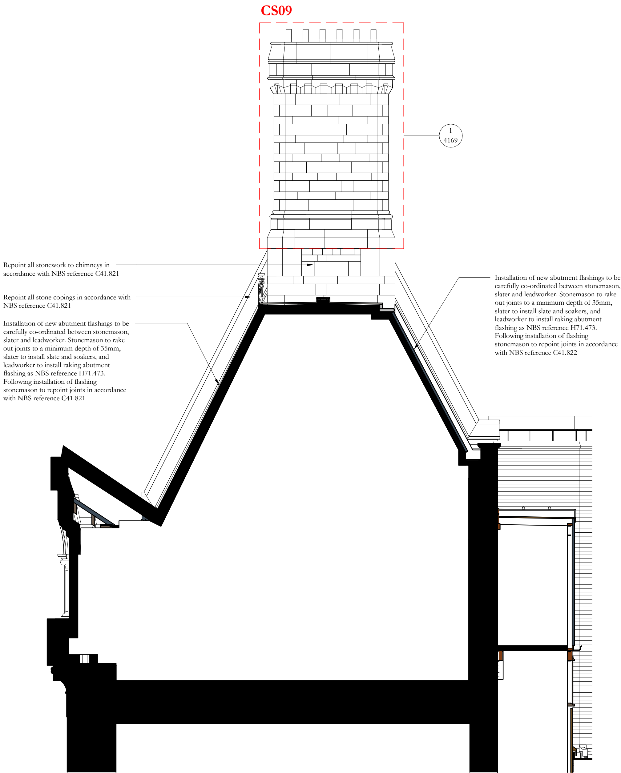
Section BT 1 : 50
