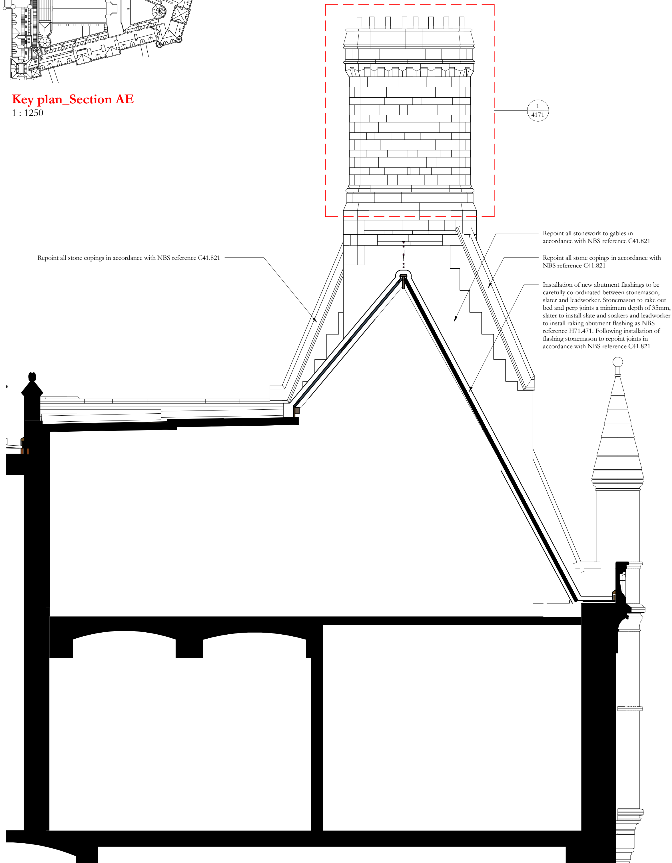
Section AE 1 : 50
