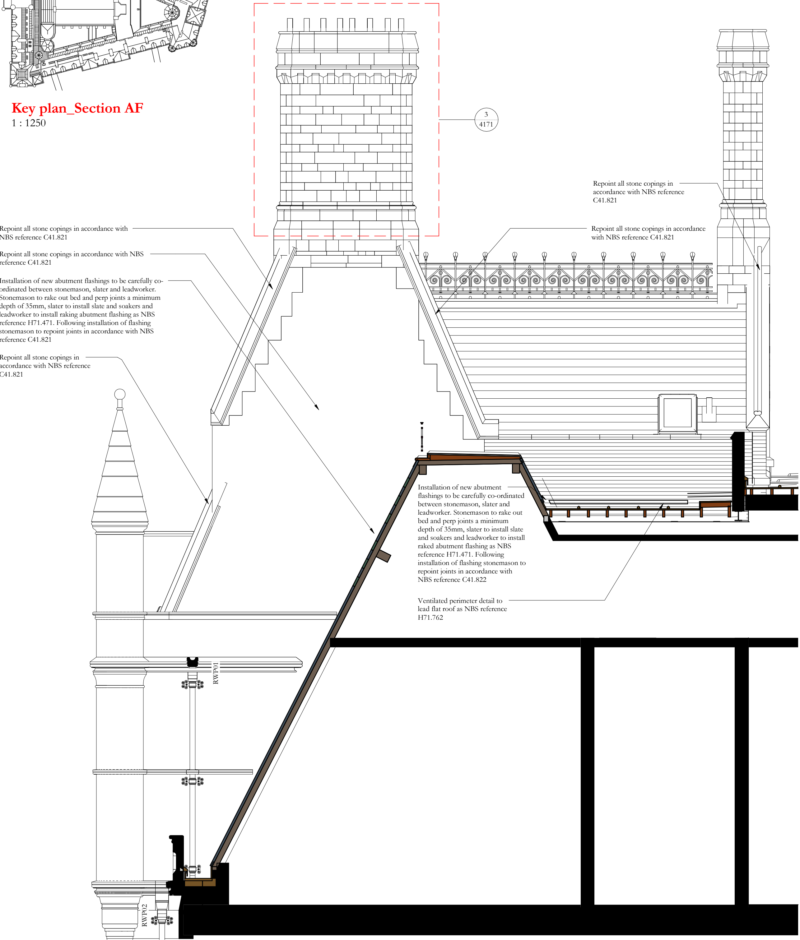
Section AF 1 : 50
