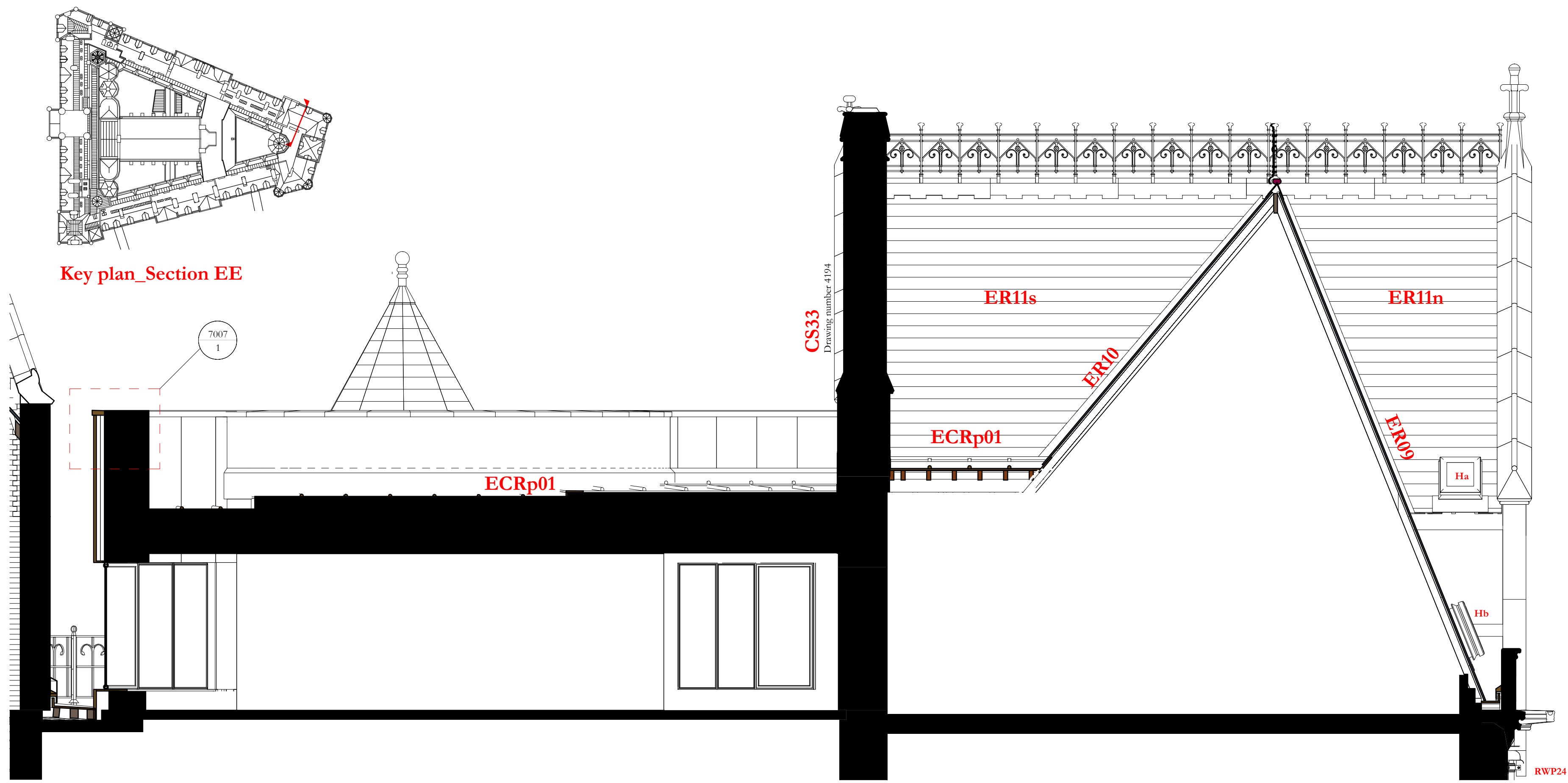
Section EE 1 : 50
