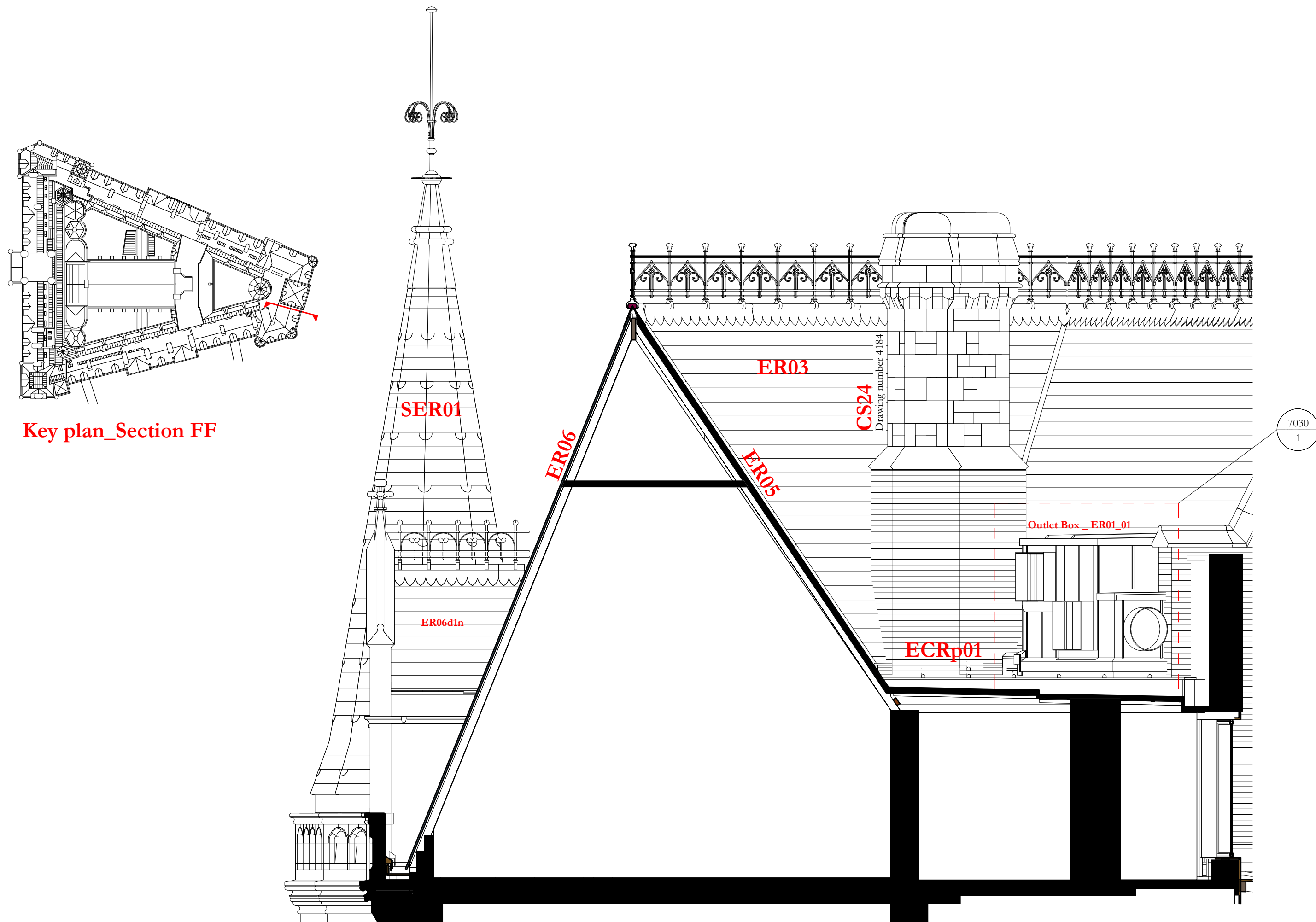
Section FF 1 : 50
