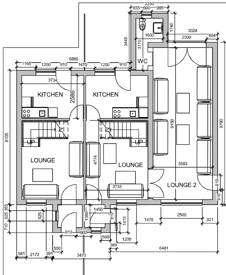
15 GROND FLOOR 1 : 100
