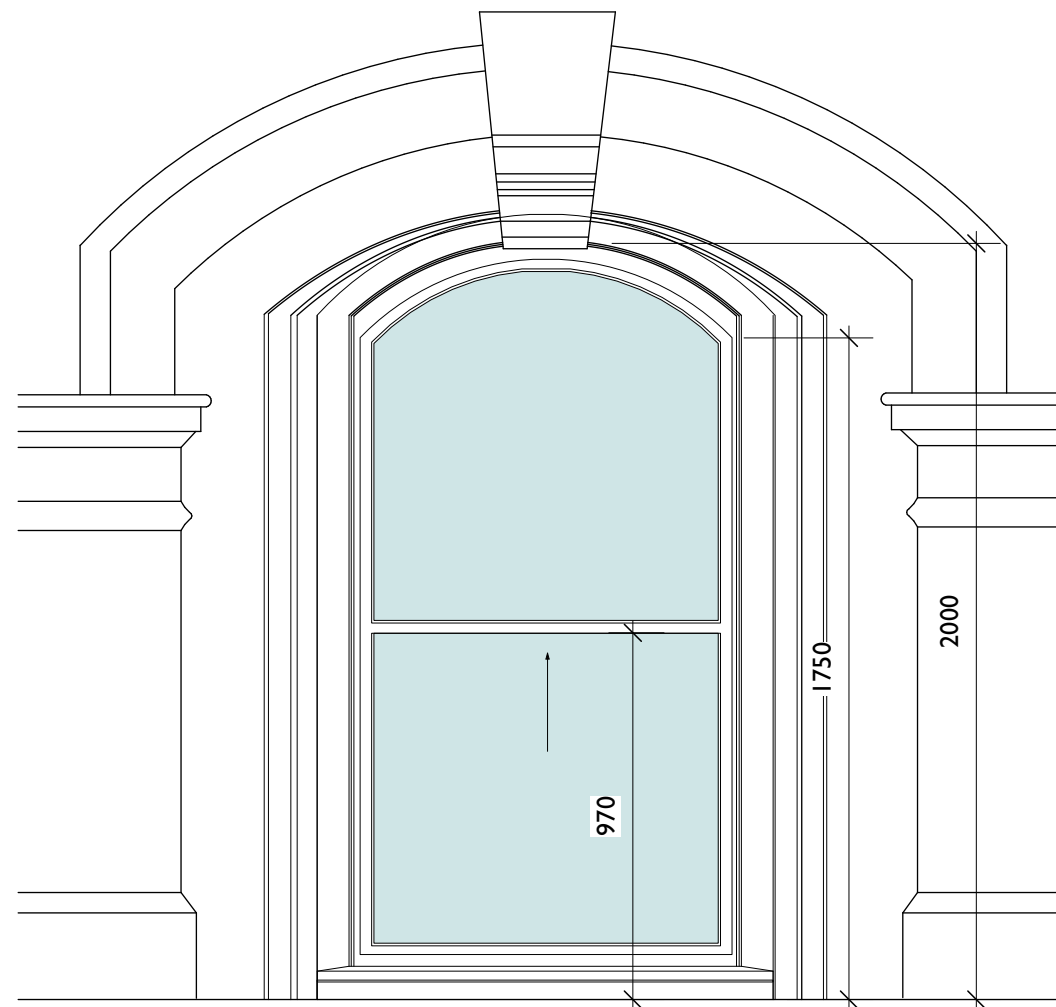
Elevation
