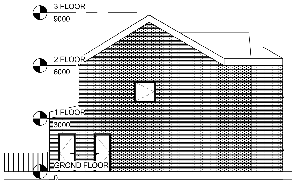
18 East 1 : 100
