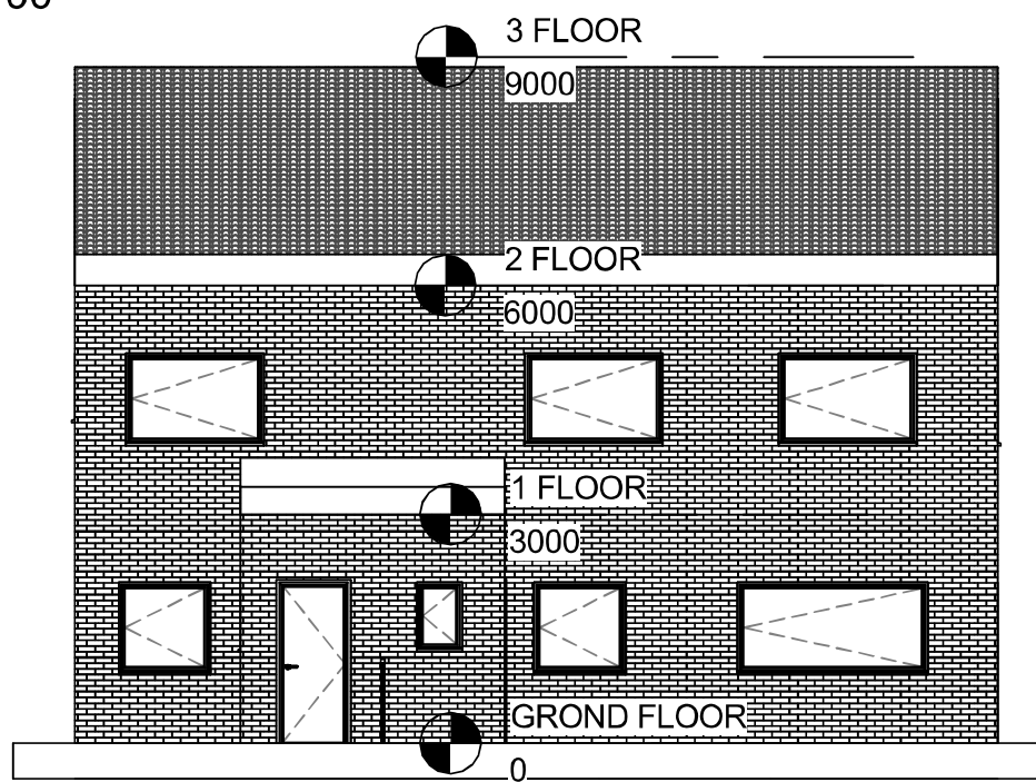
20 South 1 : 100
