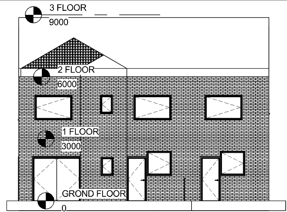
19 North 1 : 100
