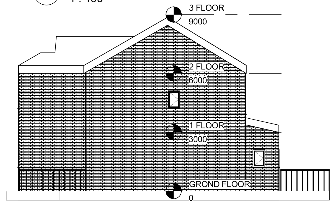
21 West 1 : 100
