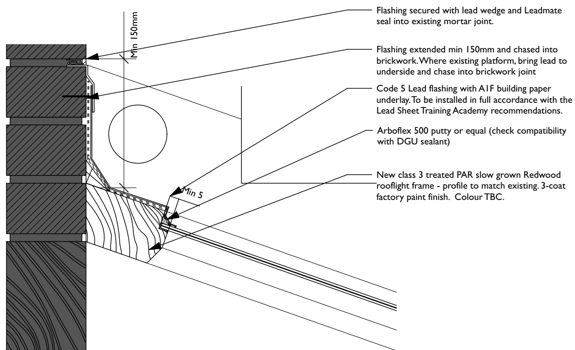
1 Jamb Detail Scale: 1:5
