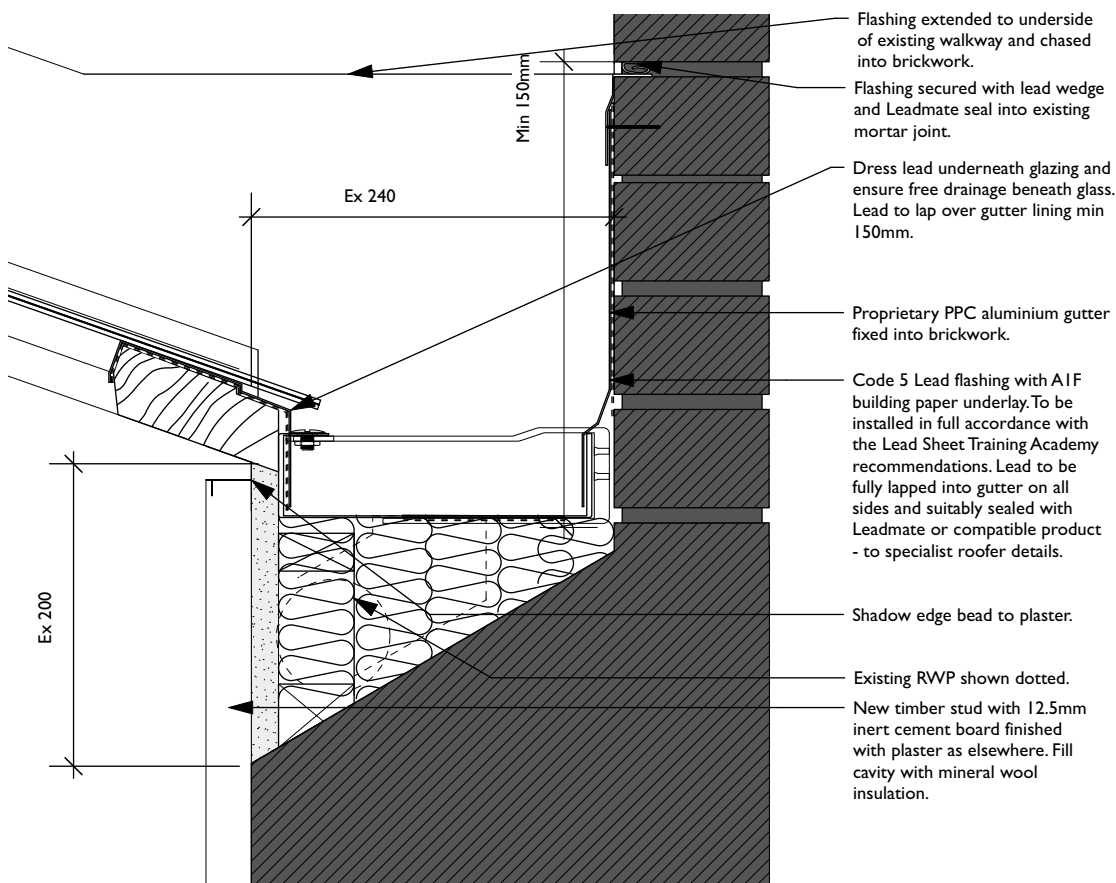
3 Base Detail Scale: 1:5
