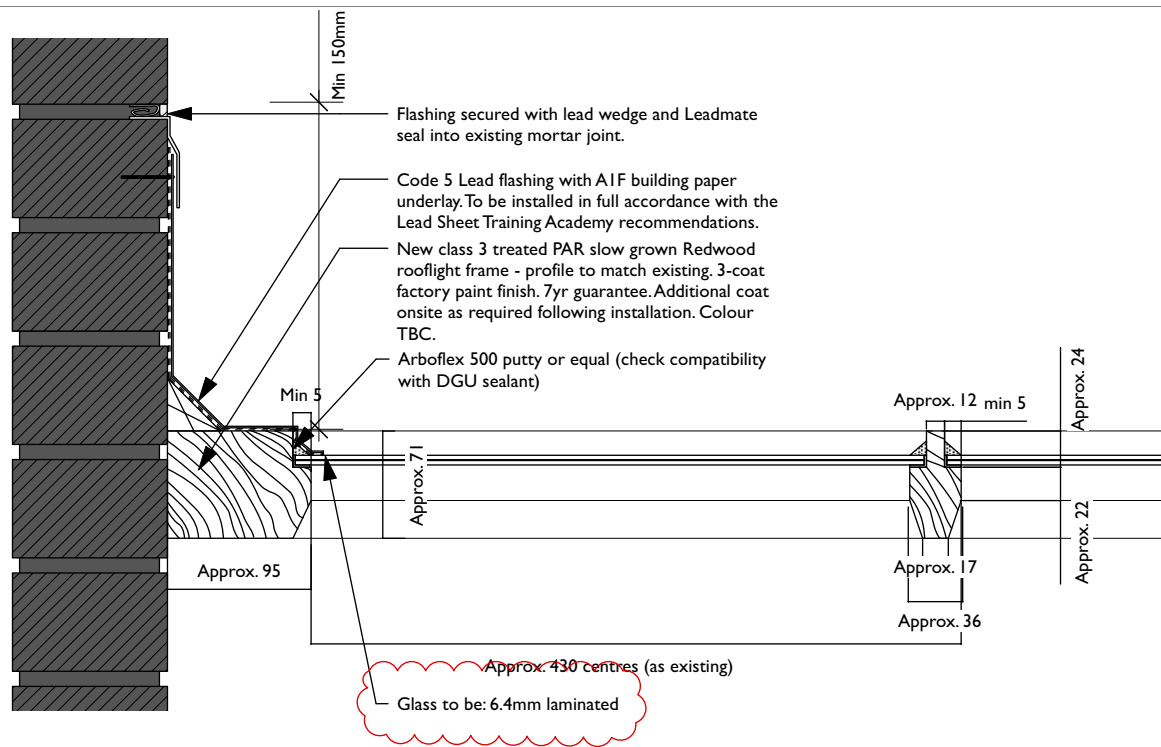
1 Jamb Detail Scale: 1:5
