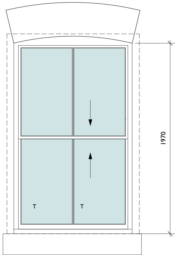
Elevation
