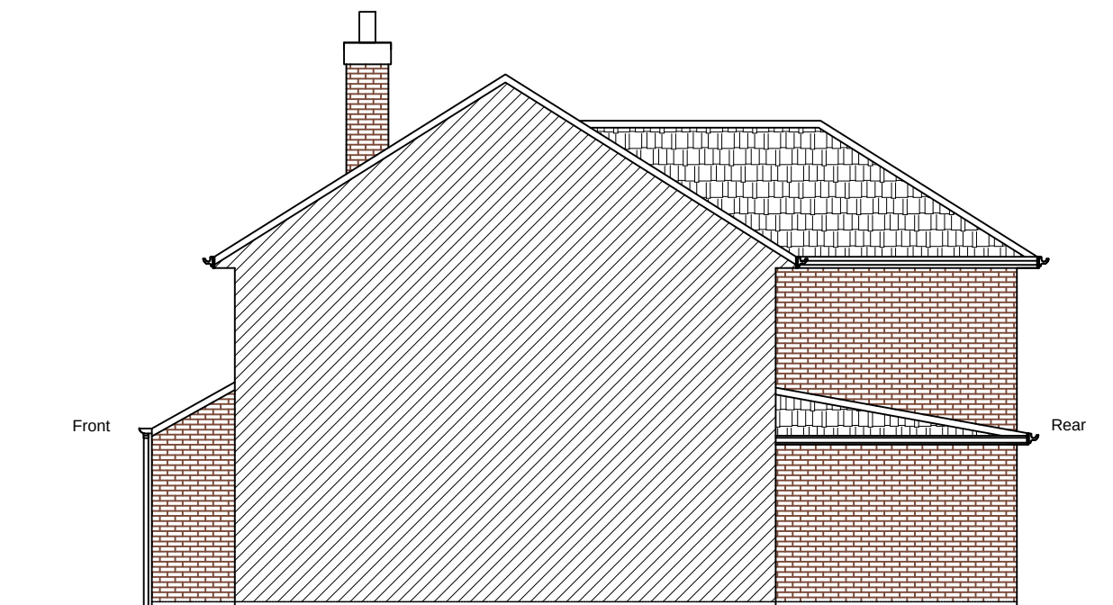
EXISTING FLANK ELEVATION
