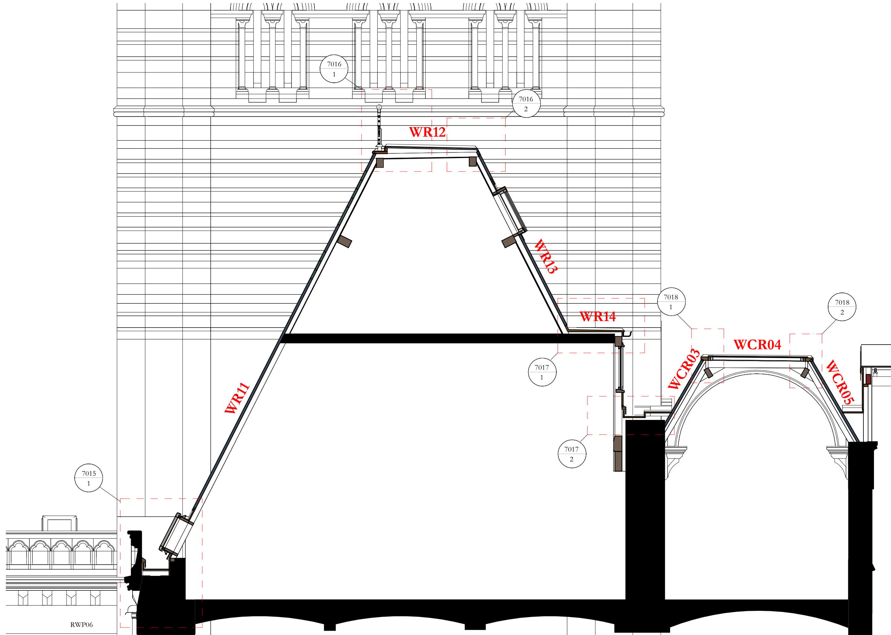
Section UU 1 : 50
