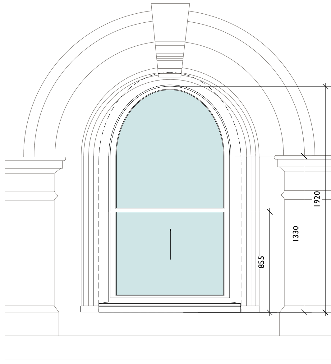
Elevation
