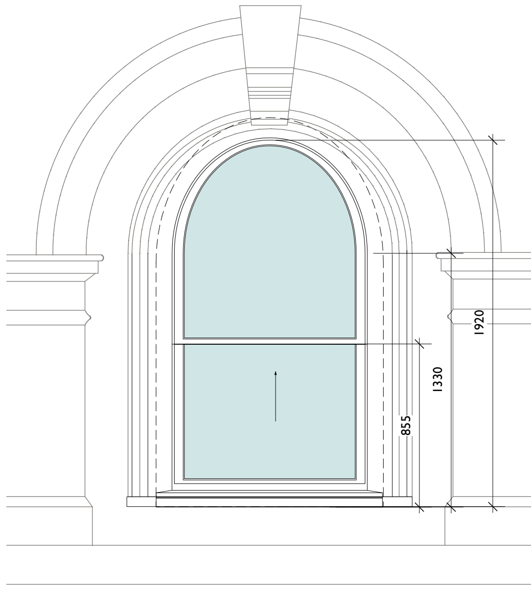
Elevation
