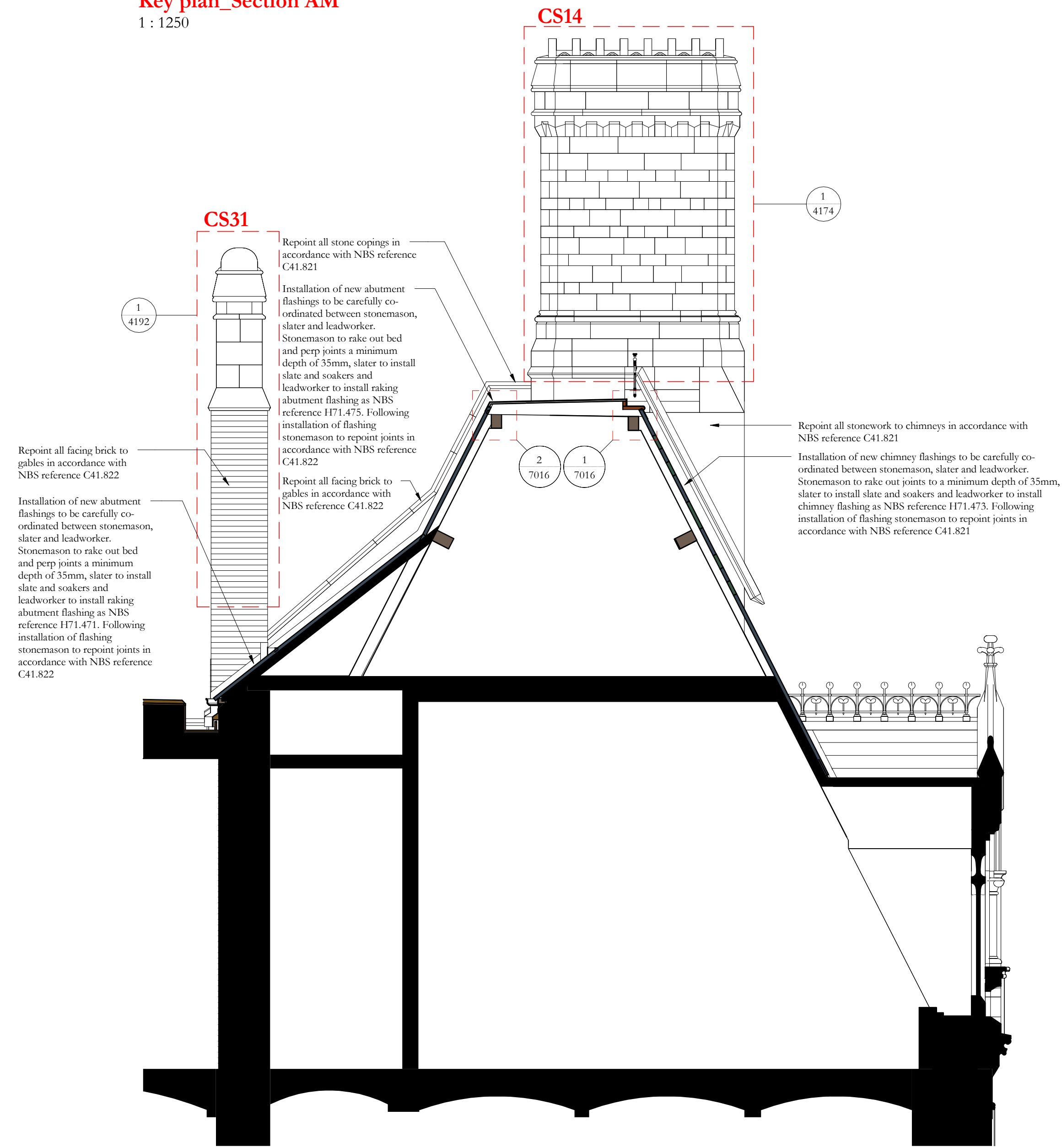
Section AM 1 : 50
