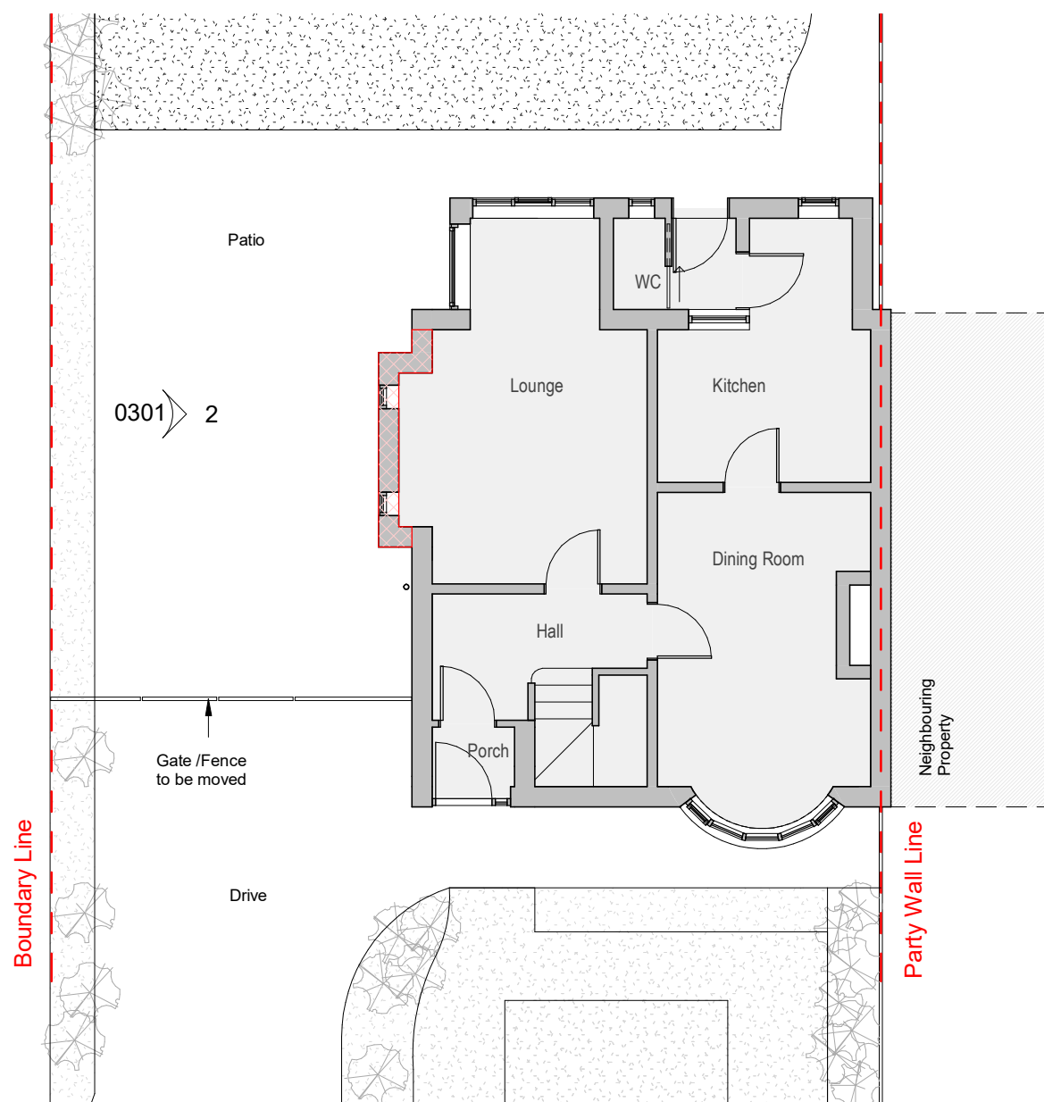
1 | Level 0_Demolition 1 : 100
