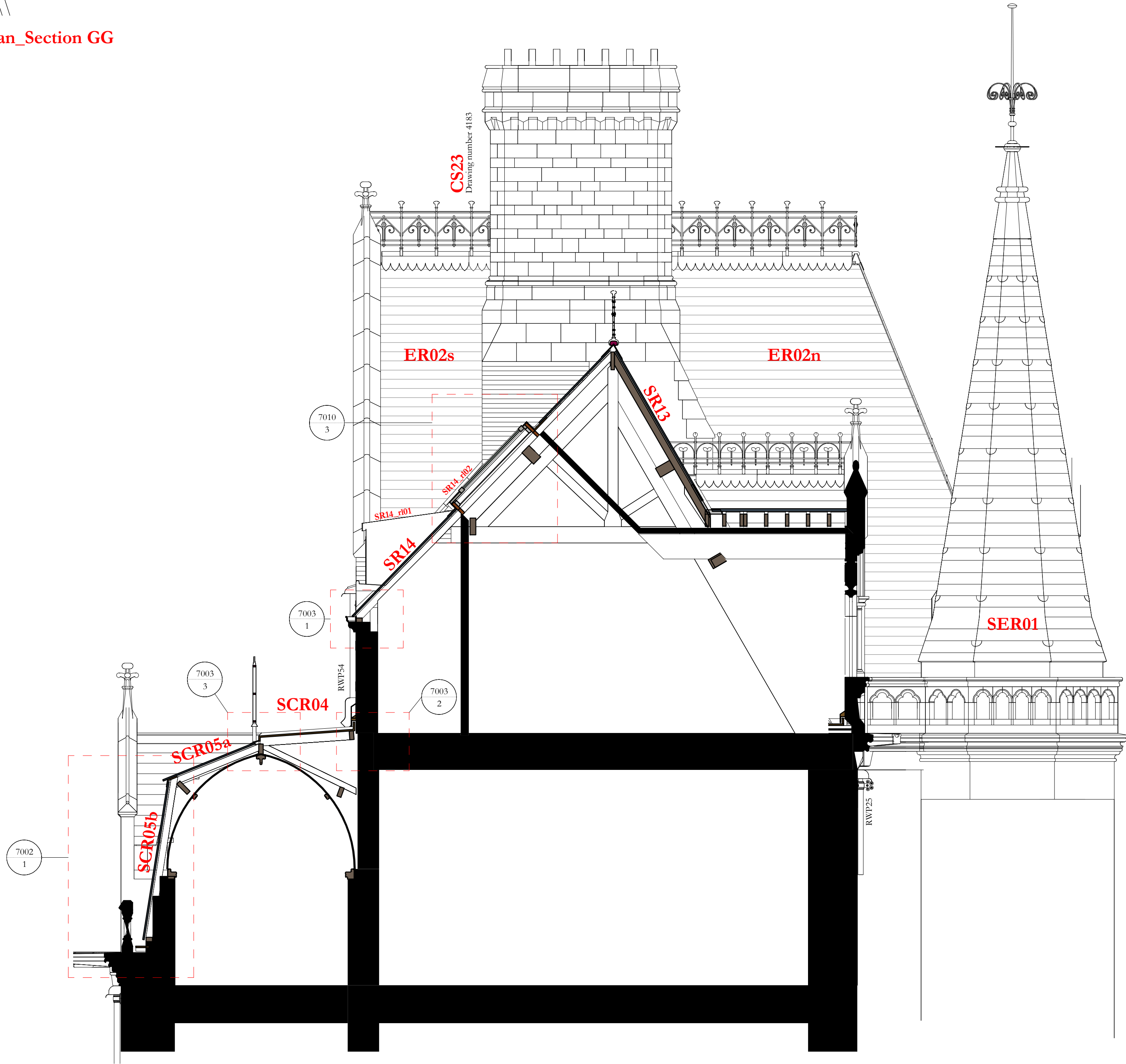
Section GG 1 : 50
