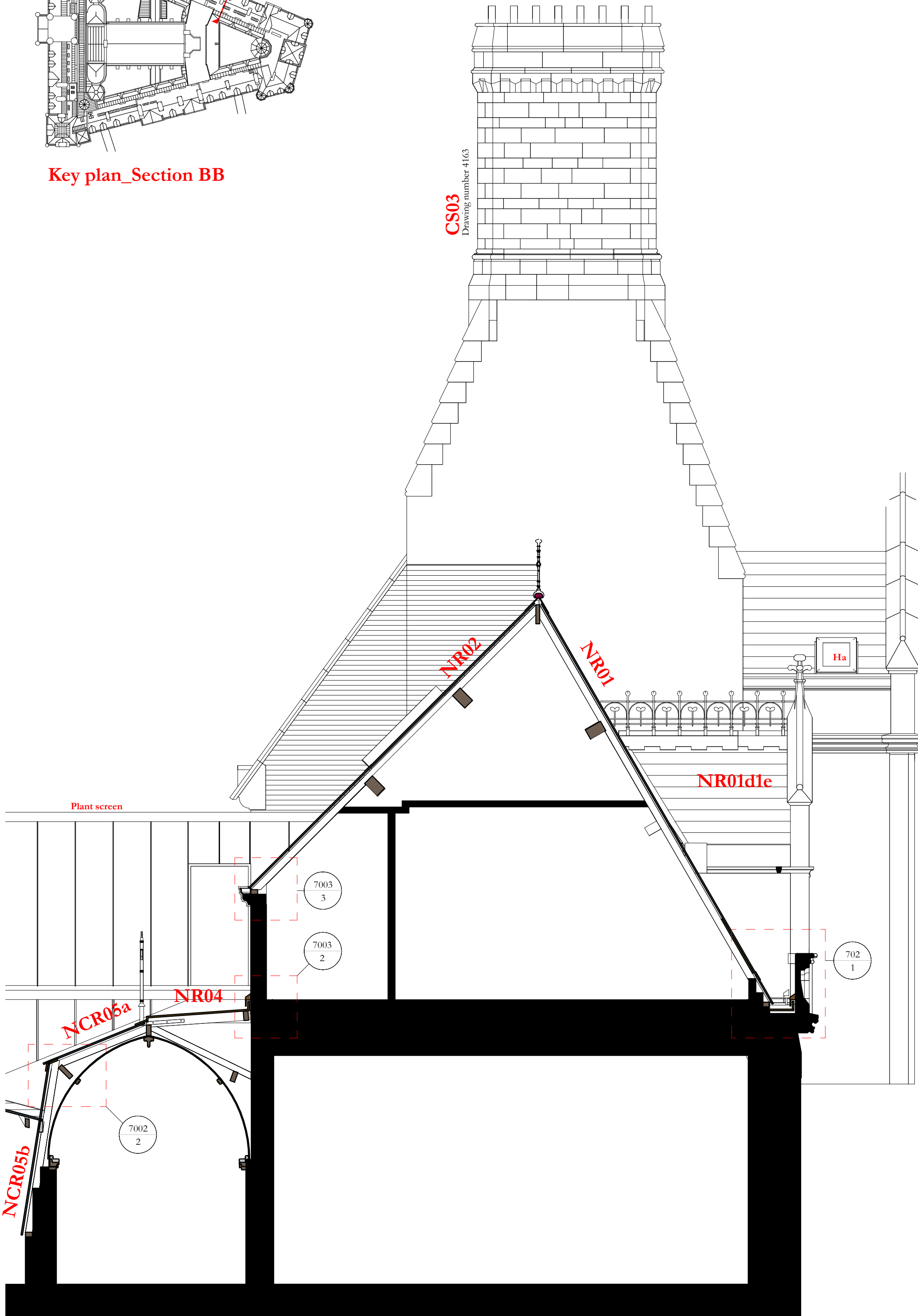
Section BB 1 : 50
