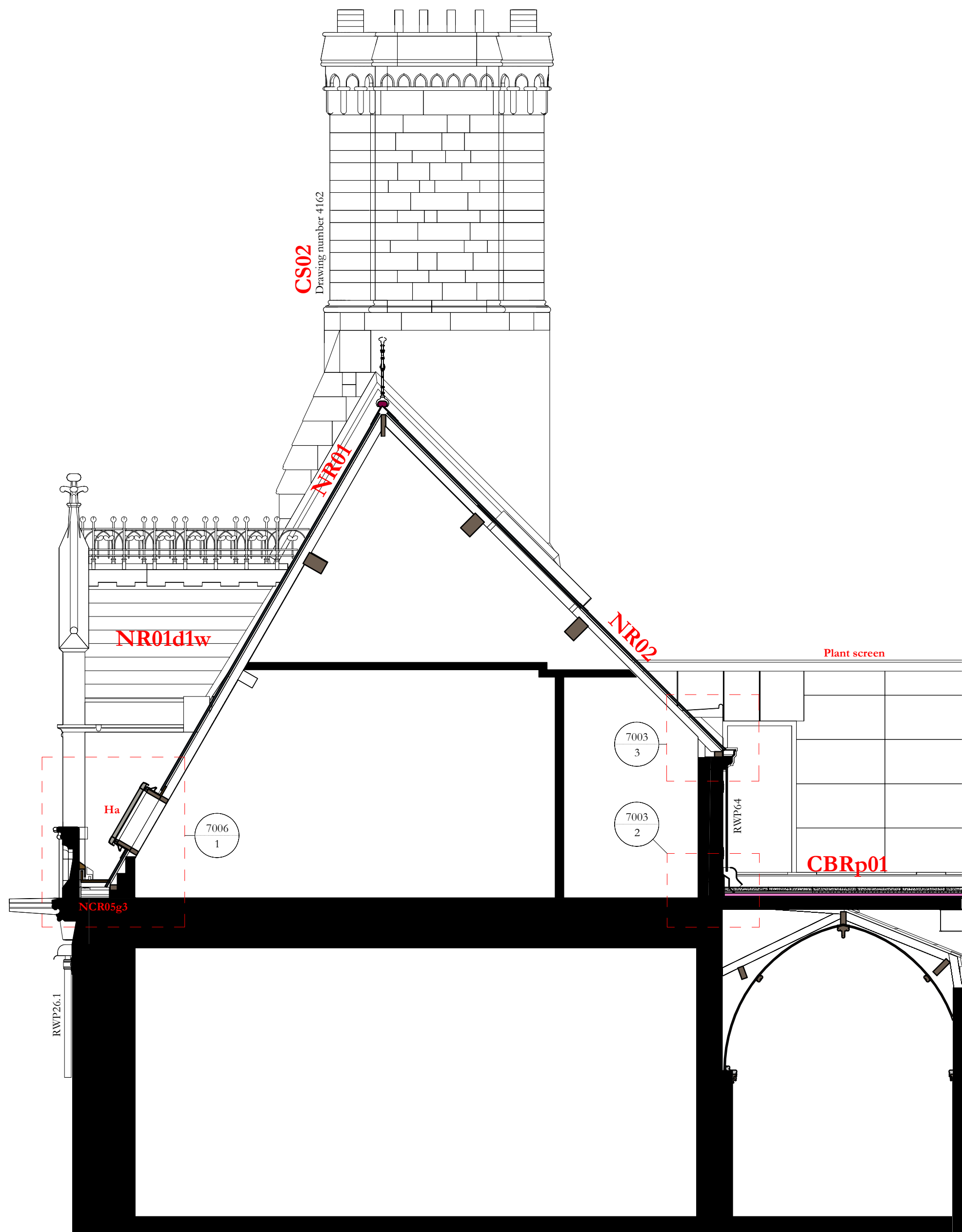
Section AA 1 : 50
