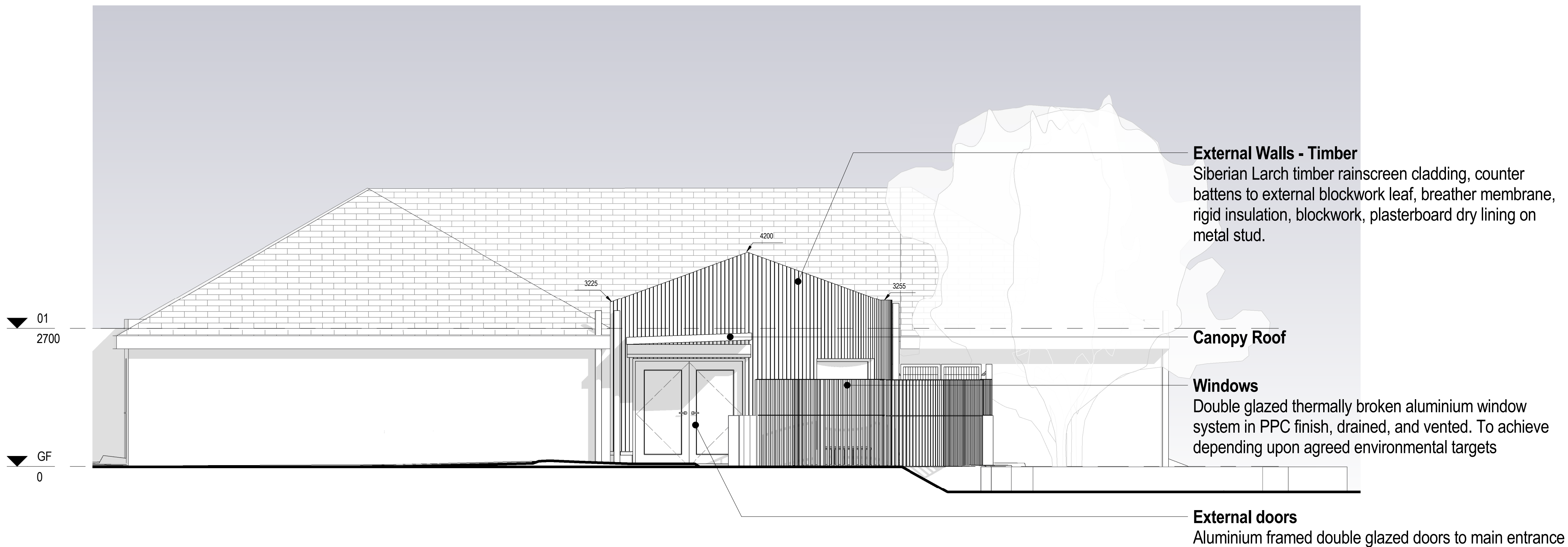
B Option 5 - Elevation B 1 : 50
